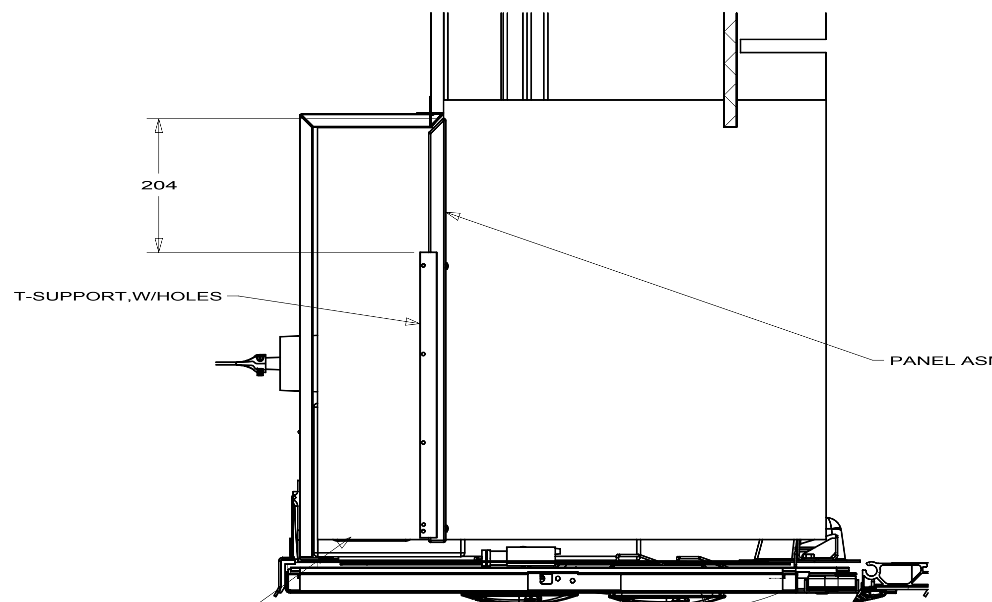
SECTION A-A (2 PLCS)
