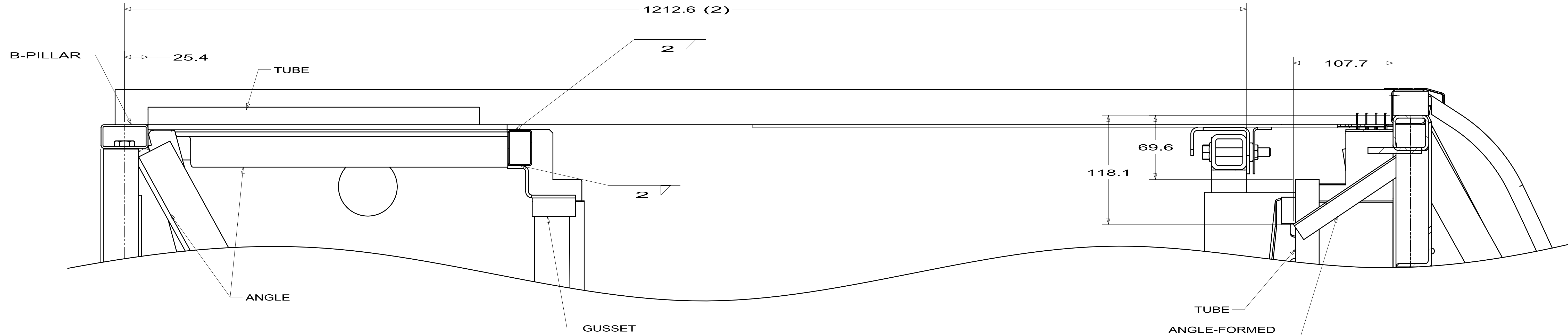
SECTION LA-LA
