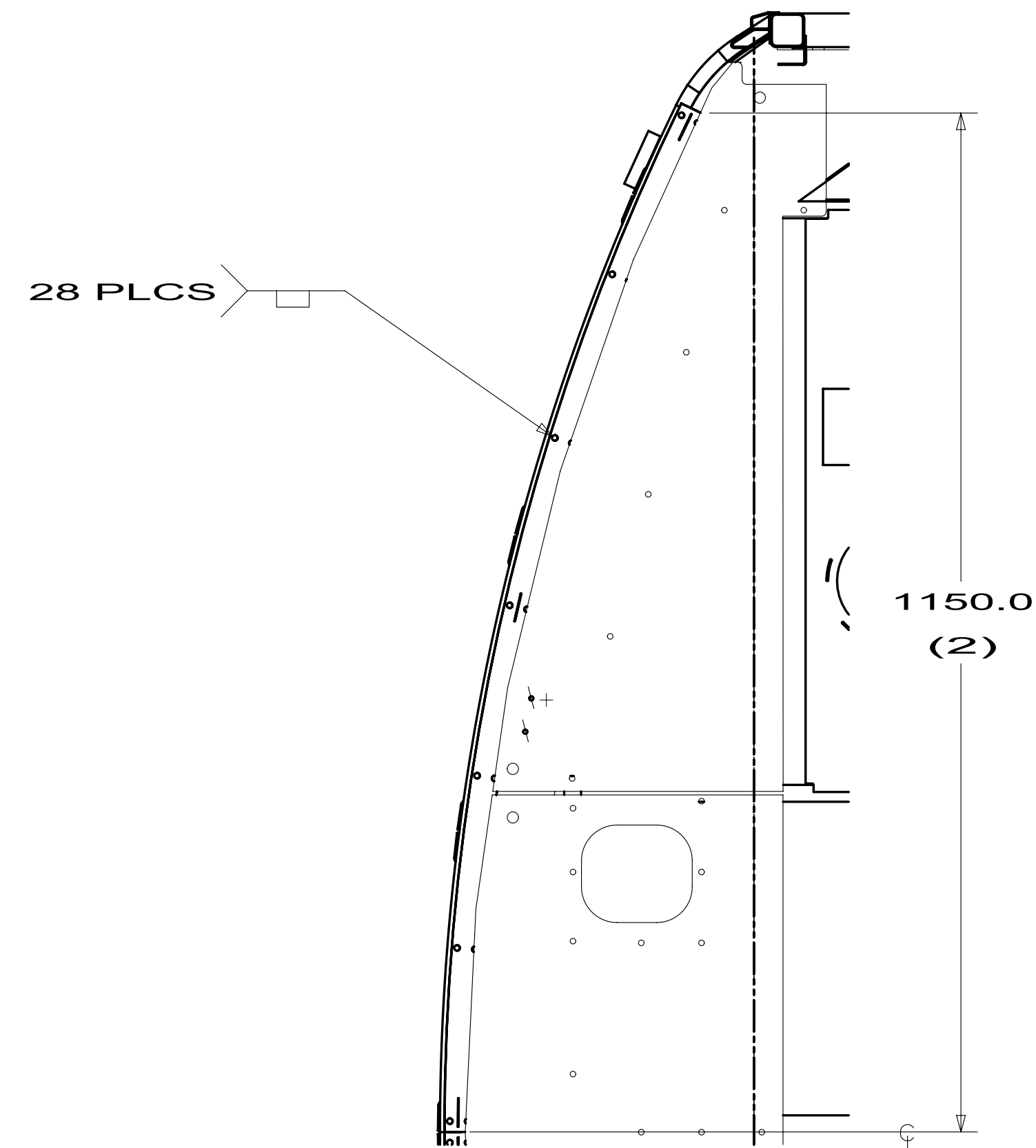
SECTION FE-FE
