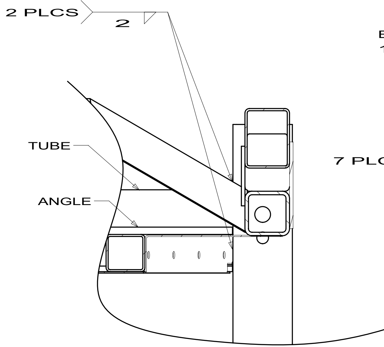
SECTION DC-DC
