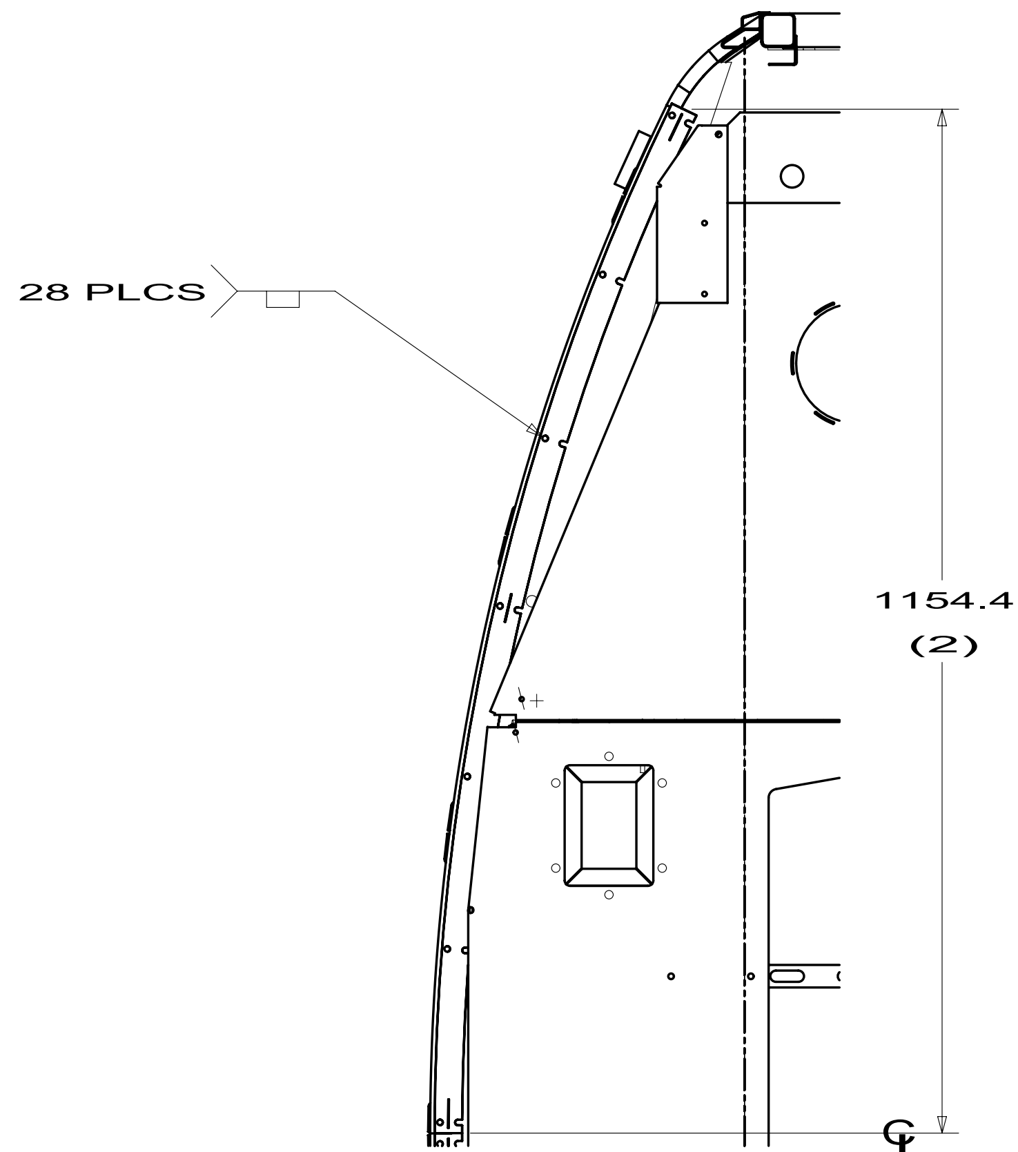
SECTION FE-FE
