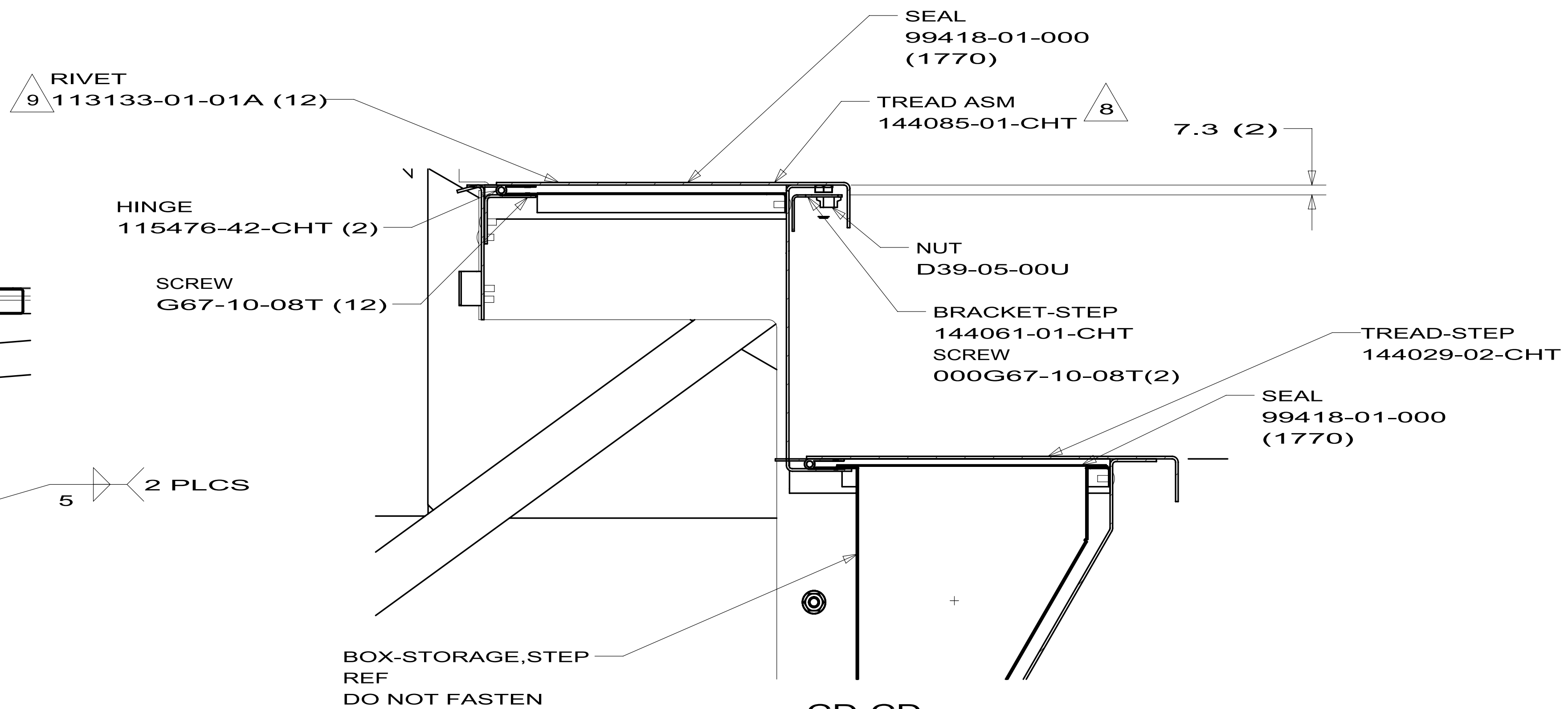
SECTION CD-CD
