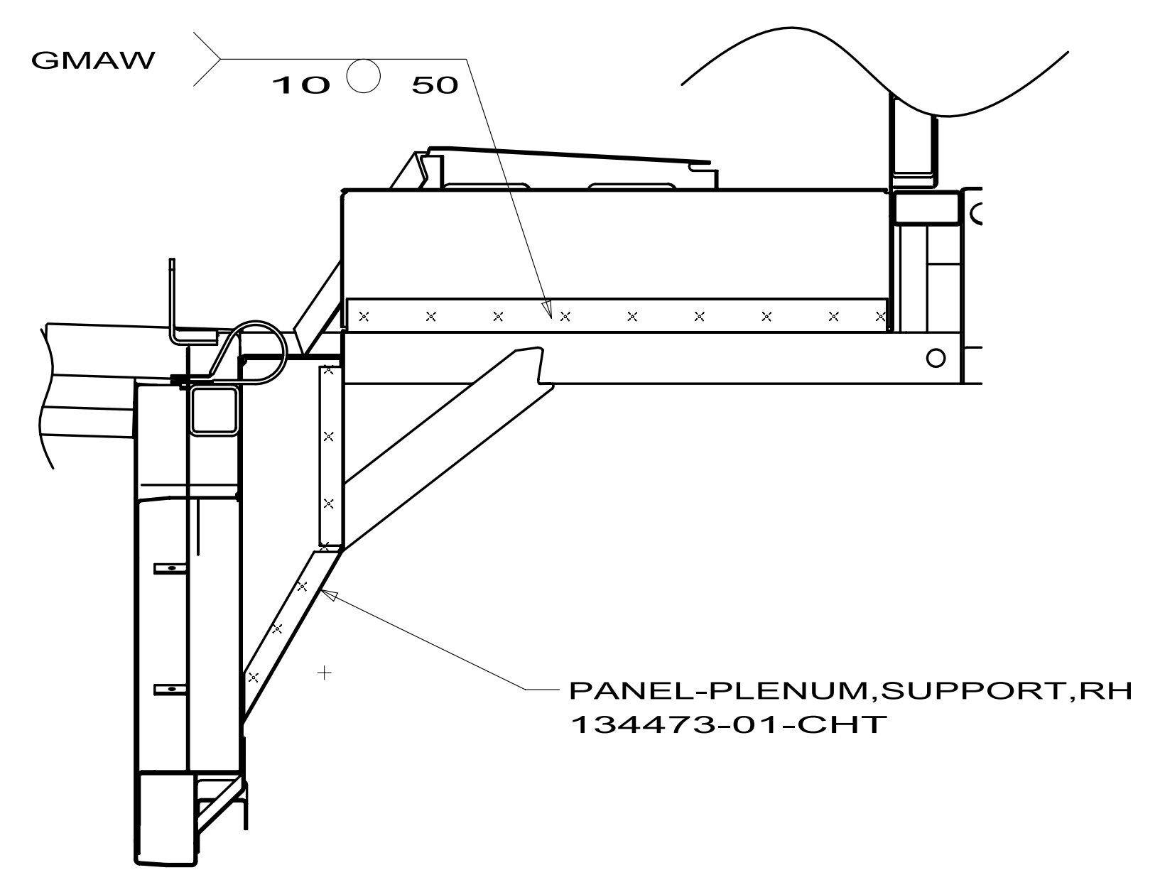
SECTION DC-DC
