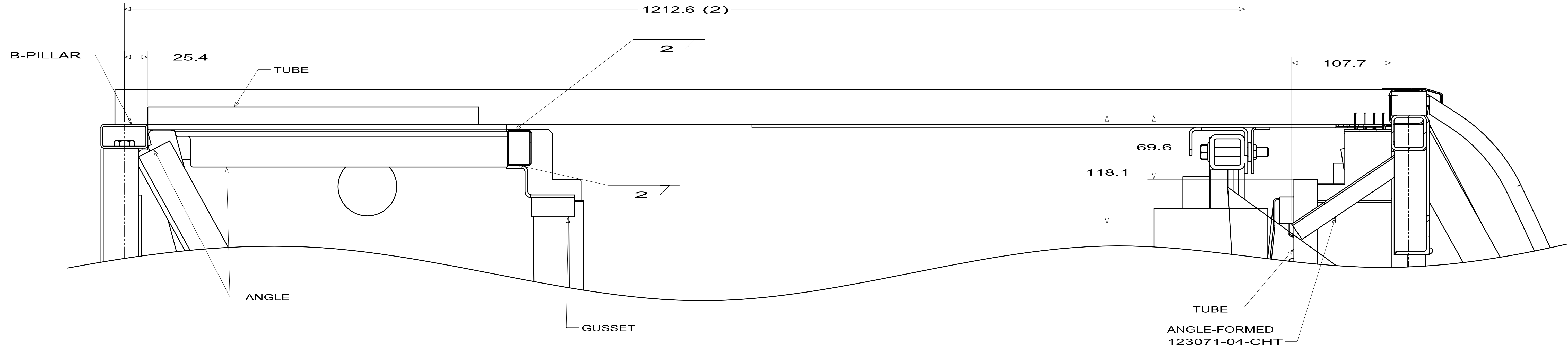
SECTION LA-LA
