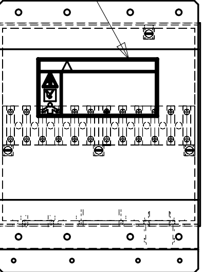
ATS SWITCH
