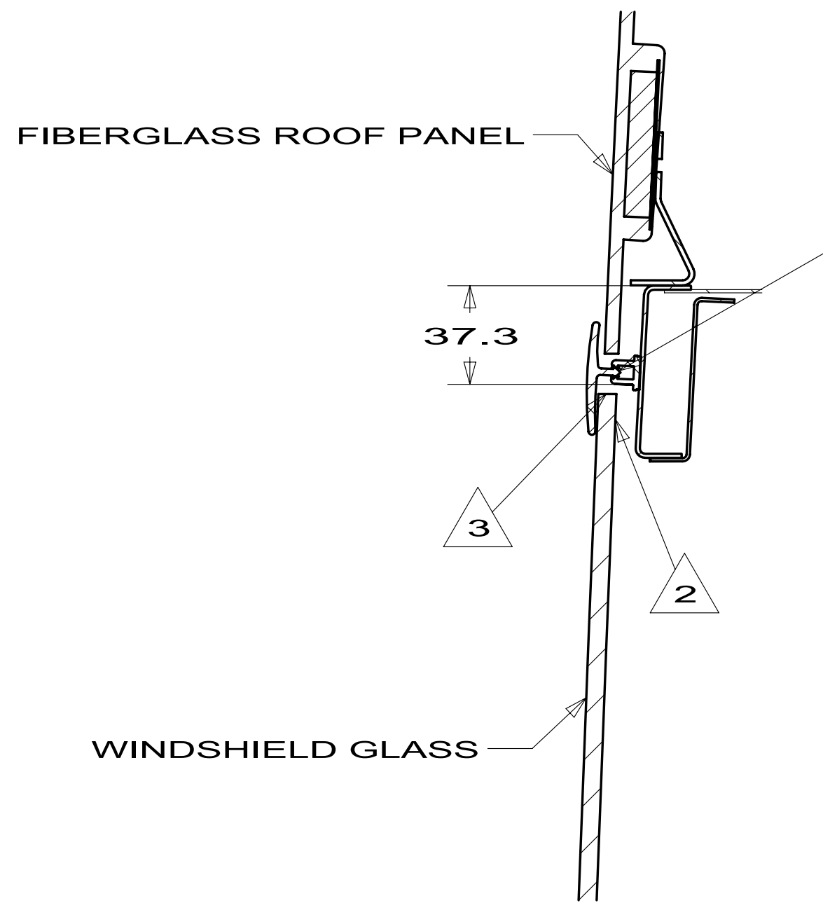
SECTION DA-DA
