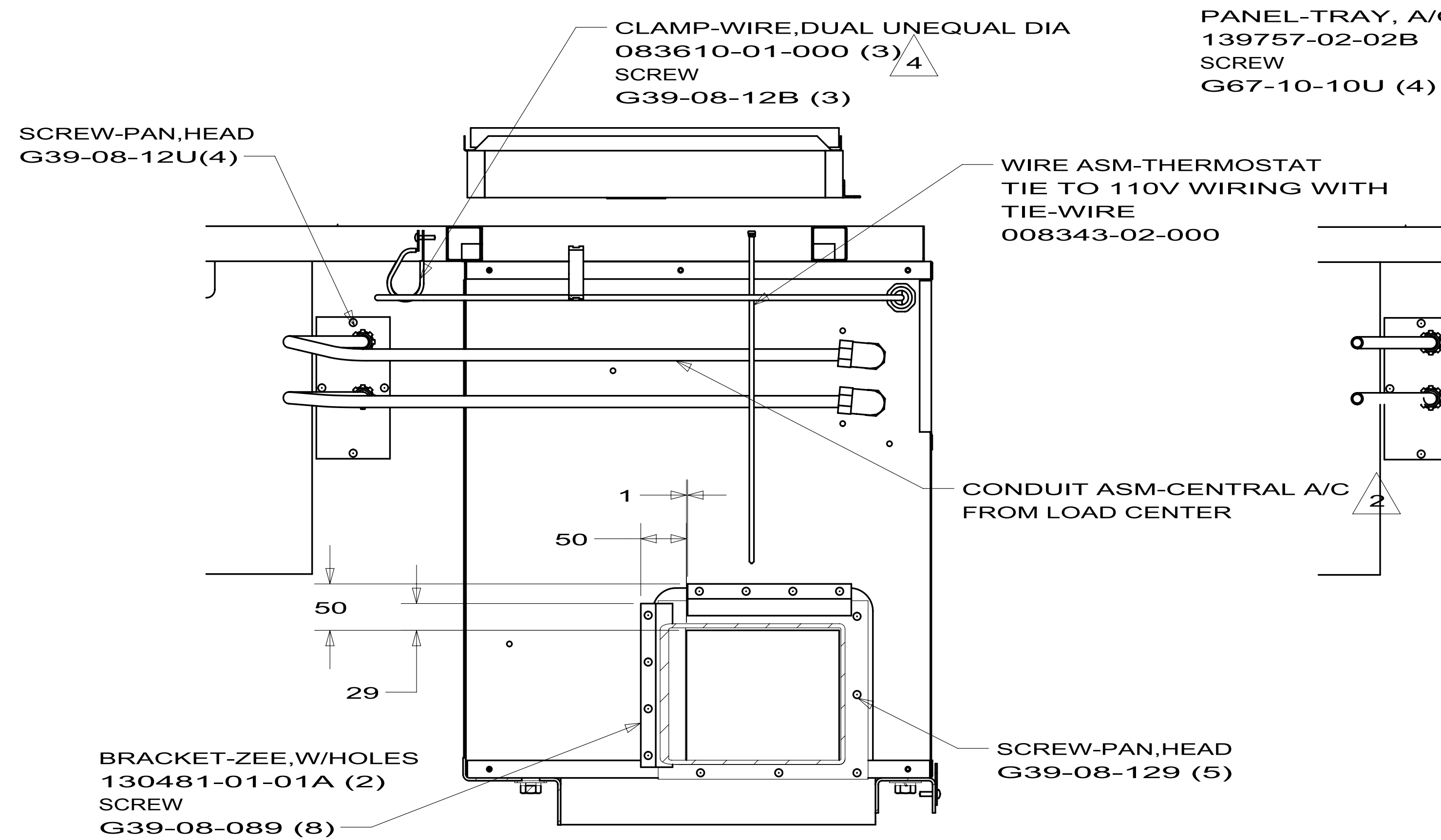
SECTION A-A
