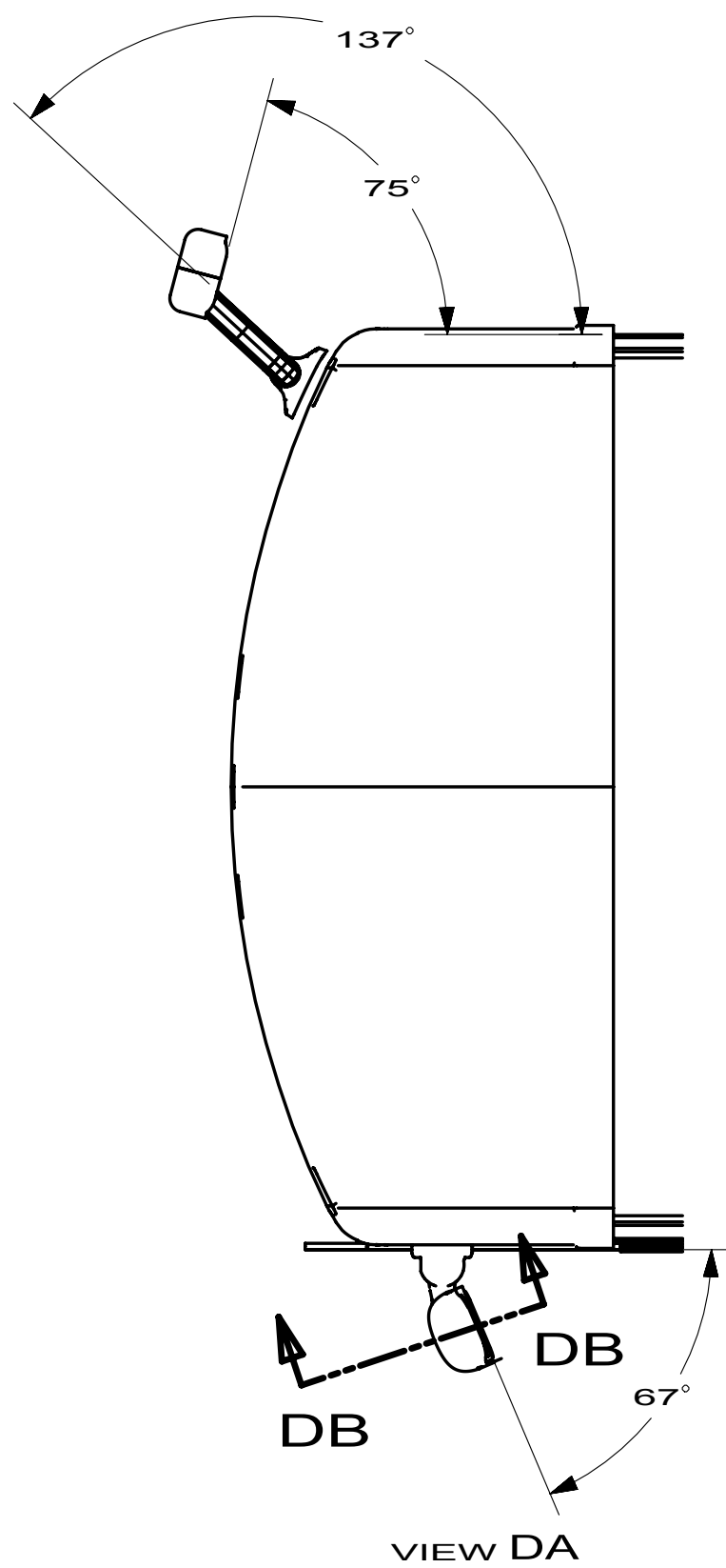
VIEW DA
