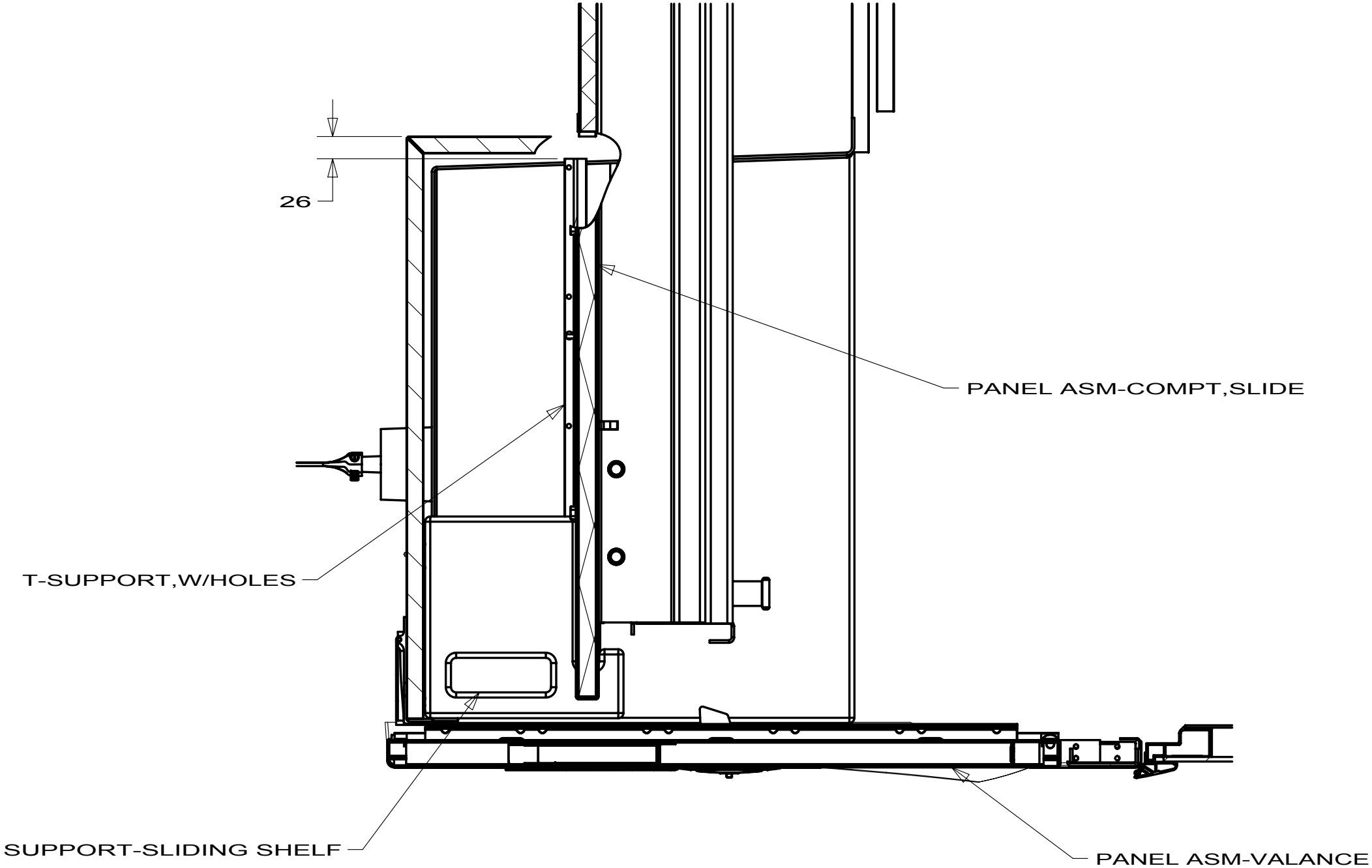
SECTION A-A
