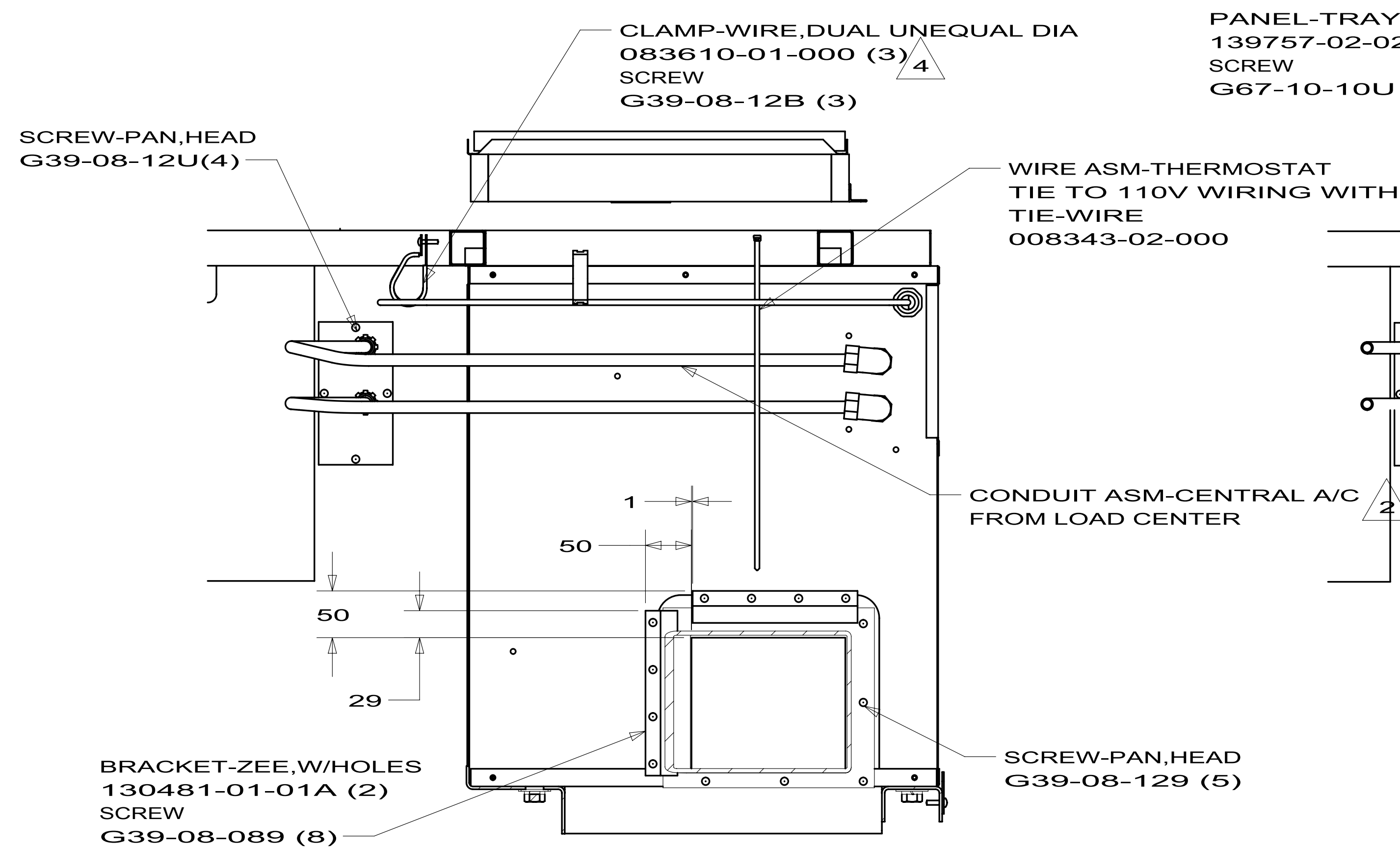
SECTION A-A
