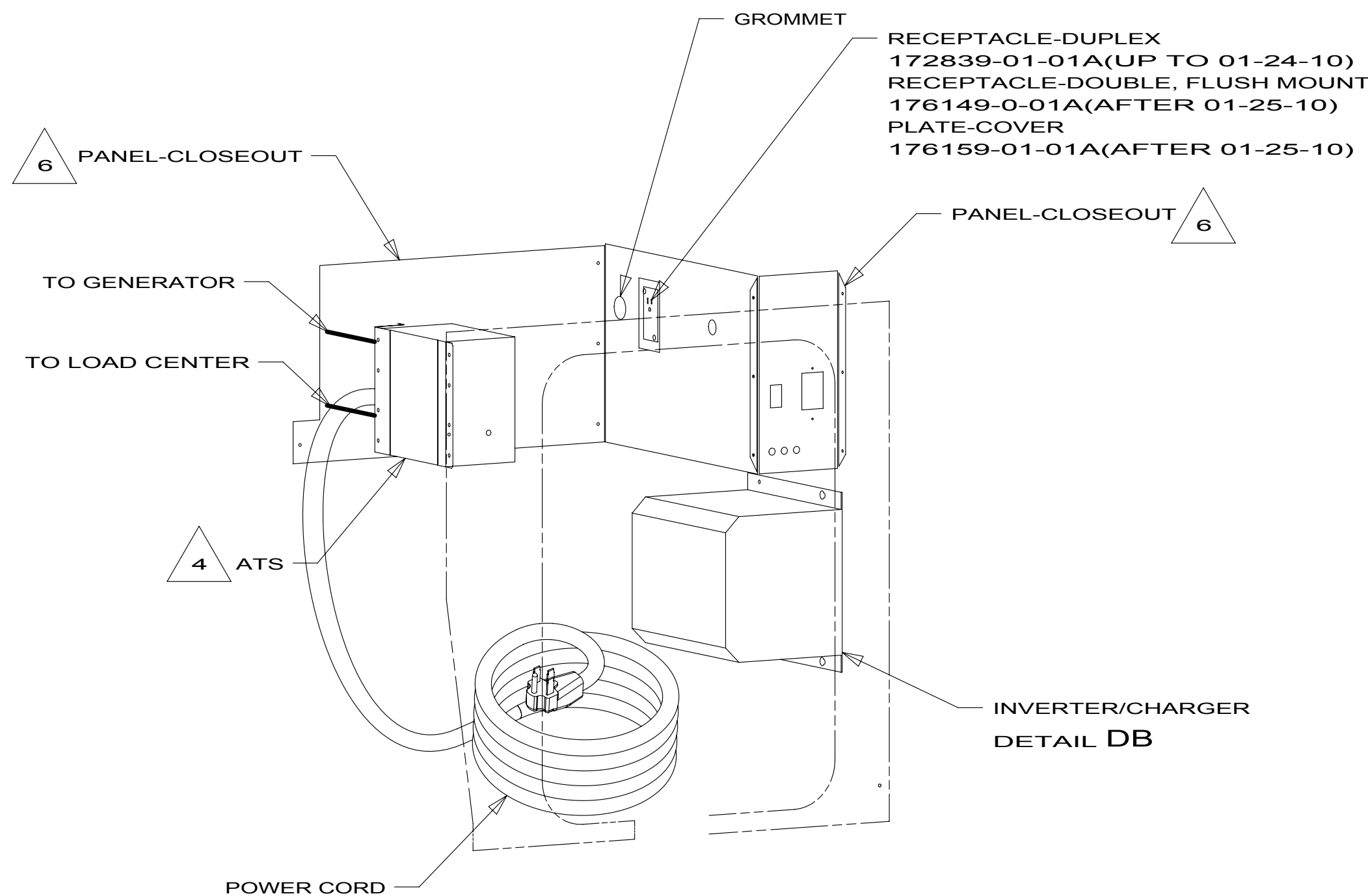
VIEW DA
