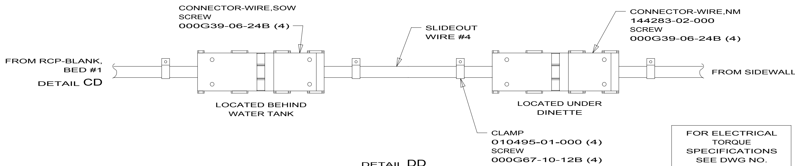
DETAIL DD
