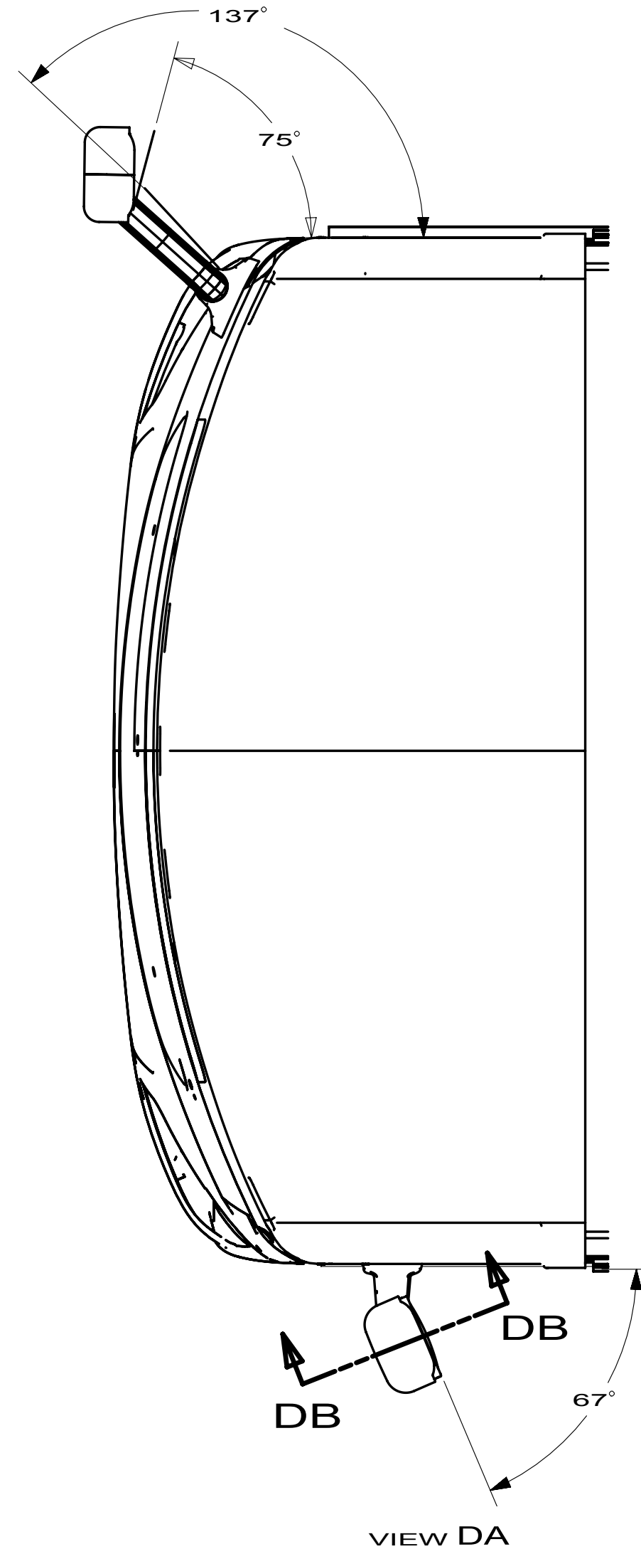
VIEW DA
