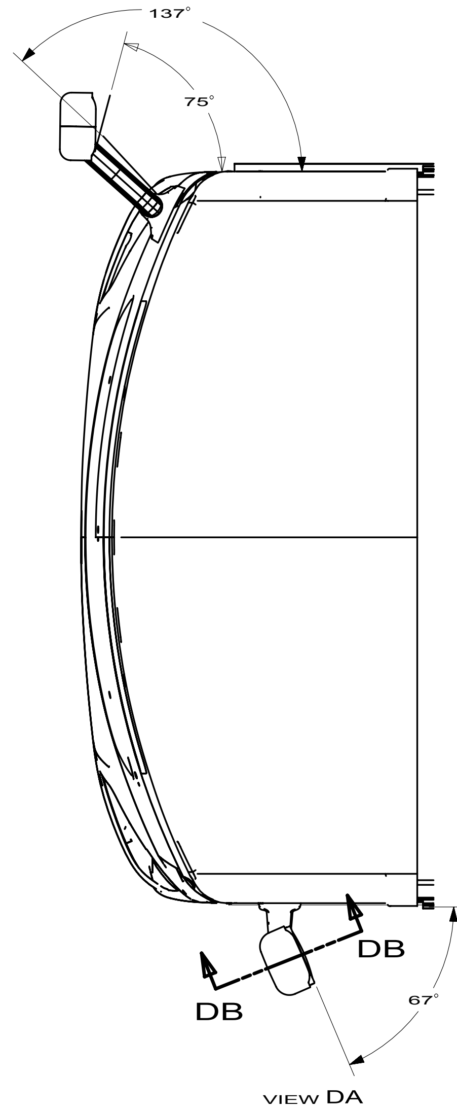
VIEW DA
