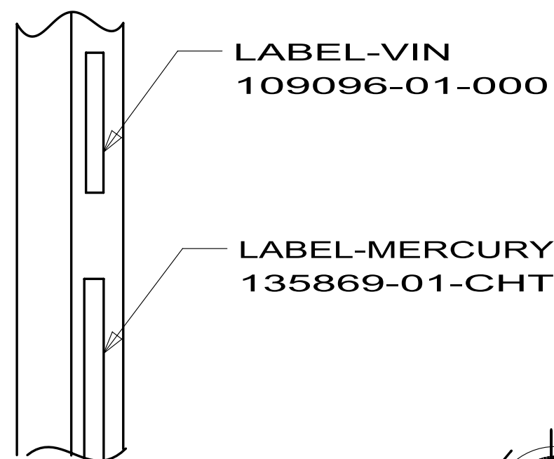
VIEW A-A
