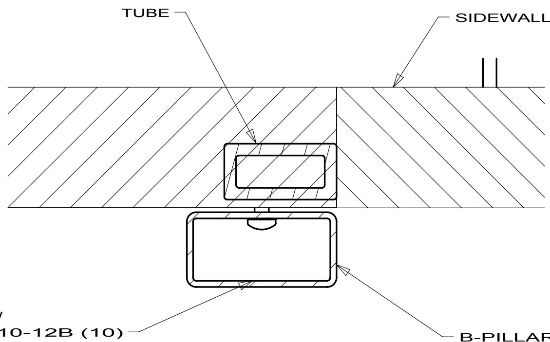
SECTION AG-AG
