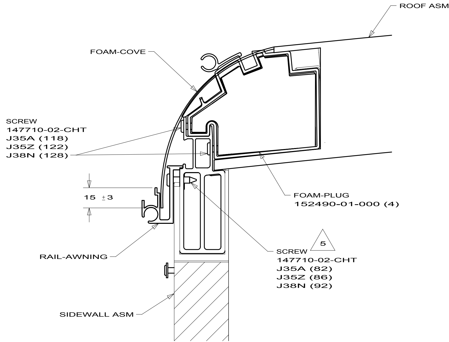
SECTION AA-AA
