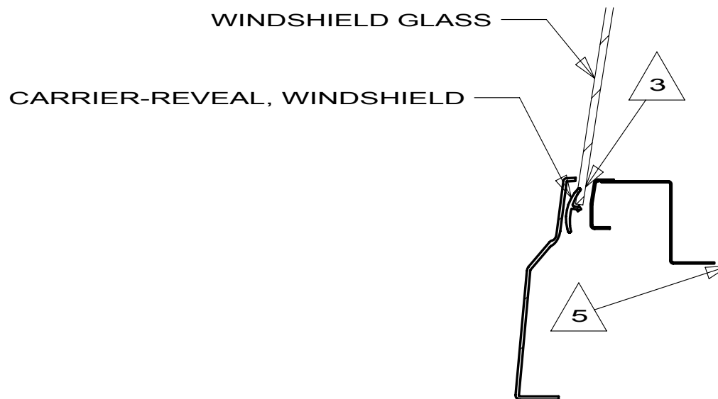
SECTION AA-AA
