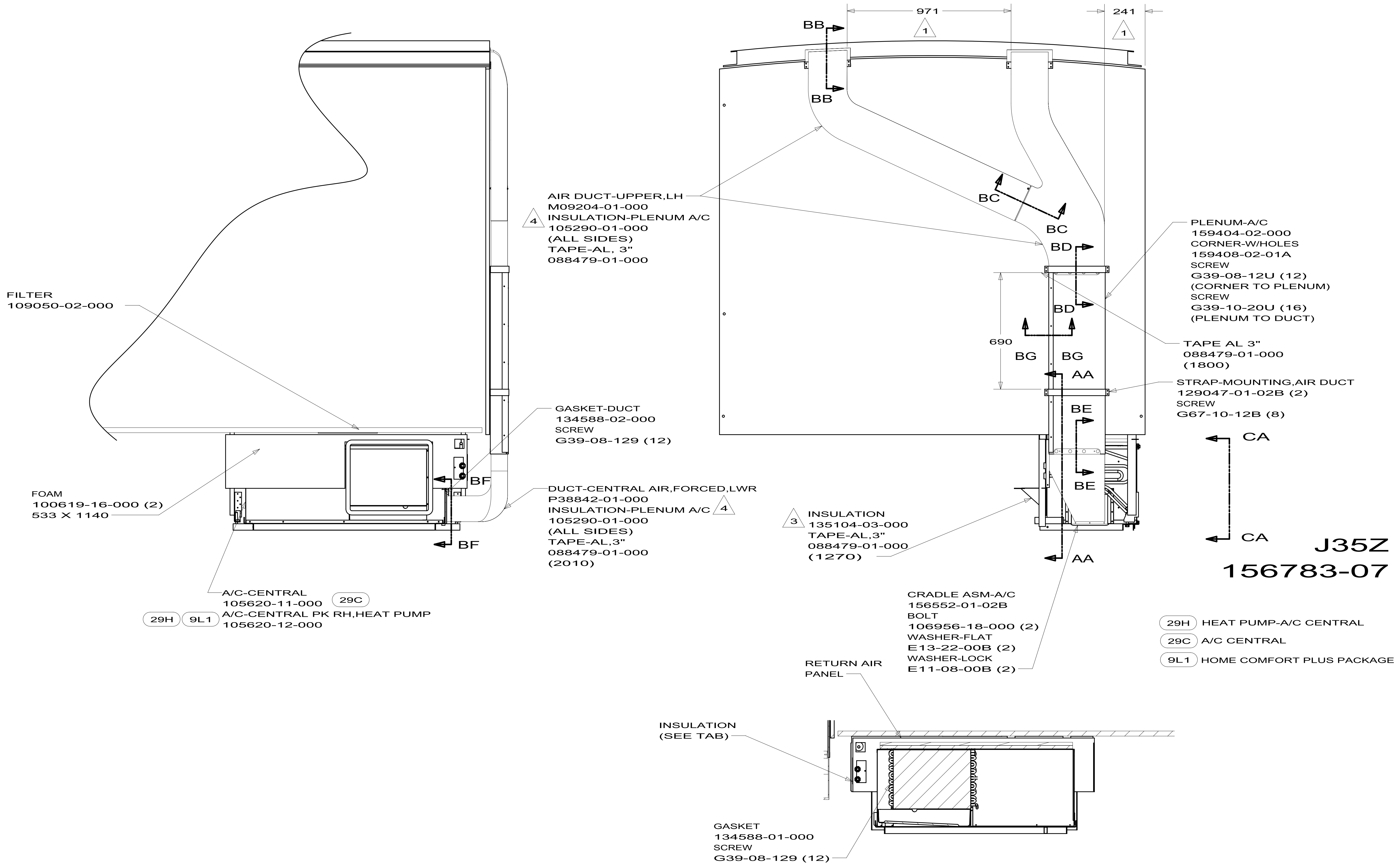
SECTION AA-AA
