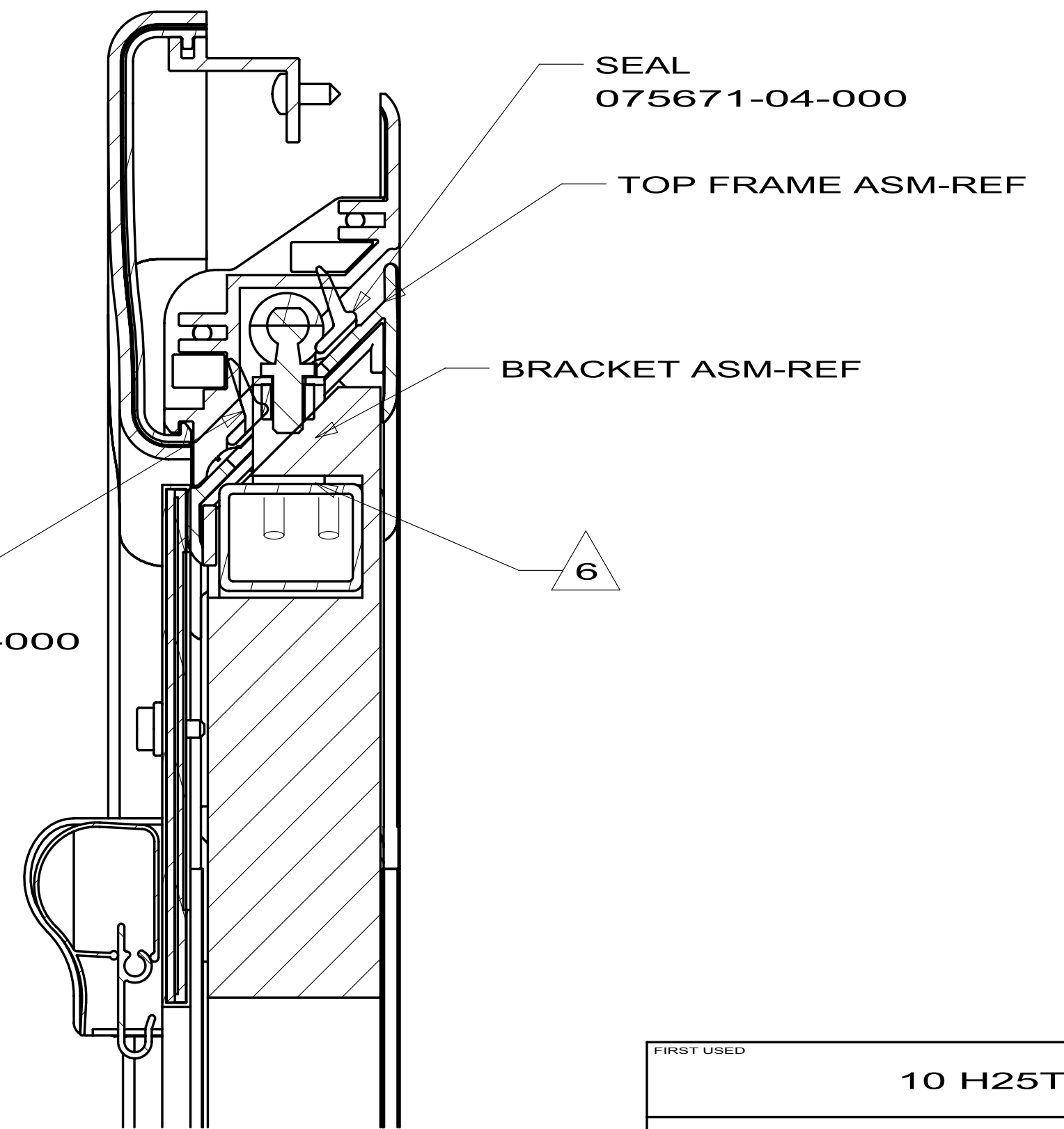
SECTION CD-CD
