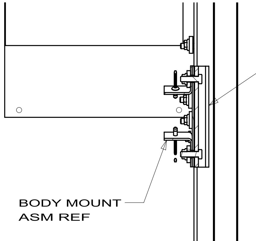
SECTION FE-FE
