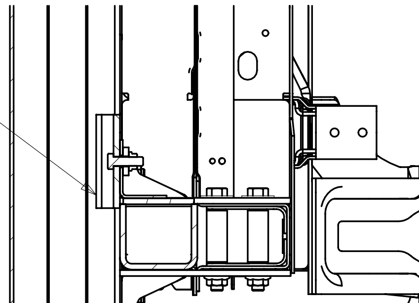
SECTION FB-FB
