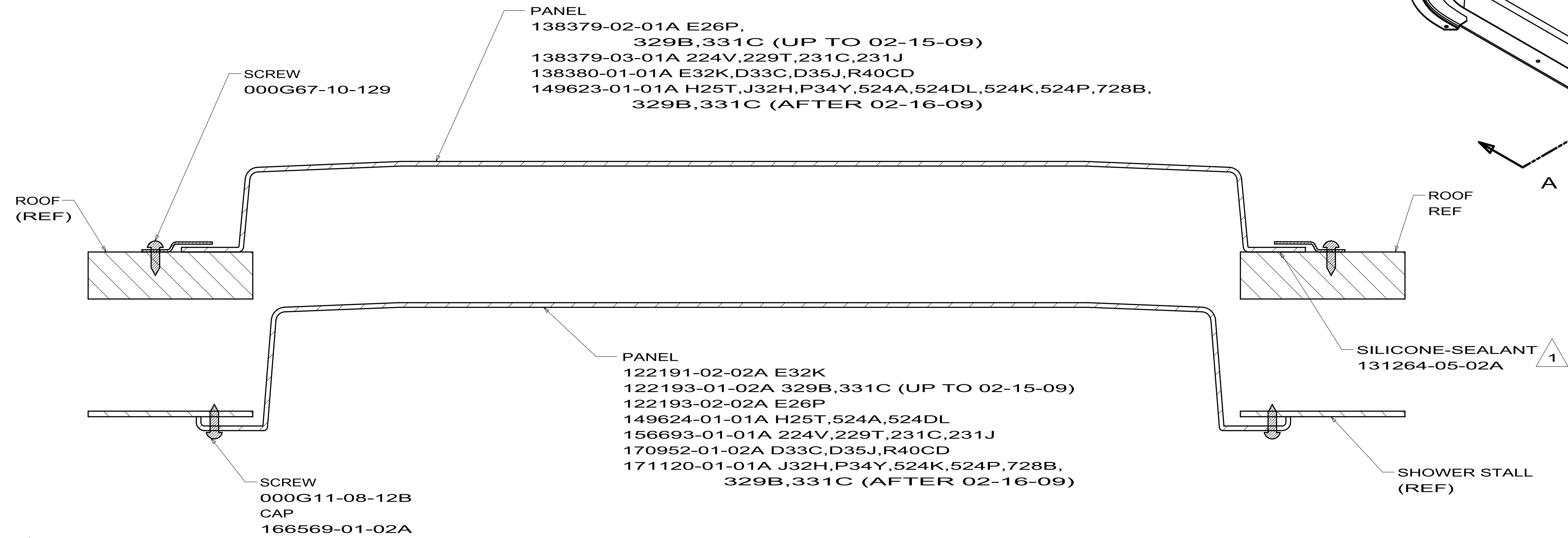
SECTION A-A
