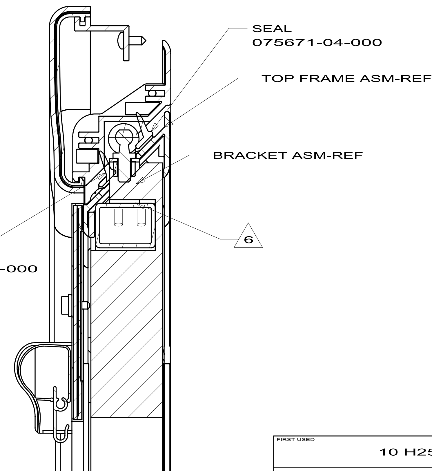
SECTION CD-CD
