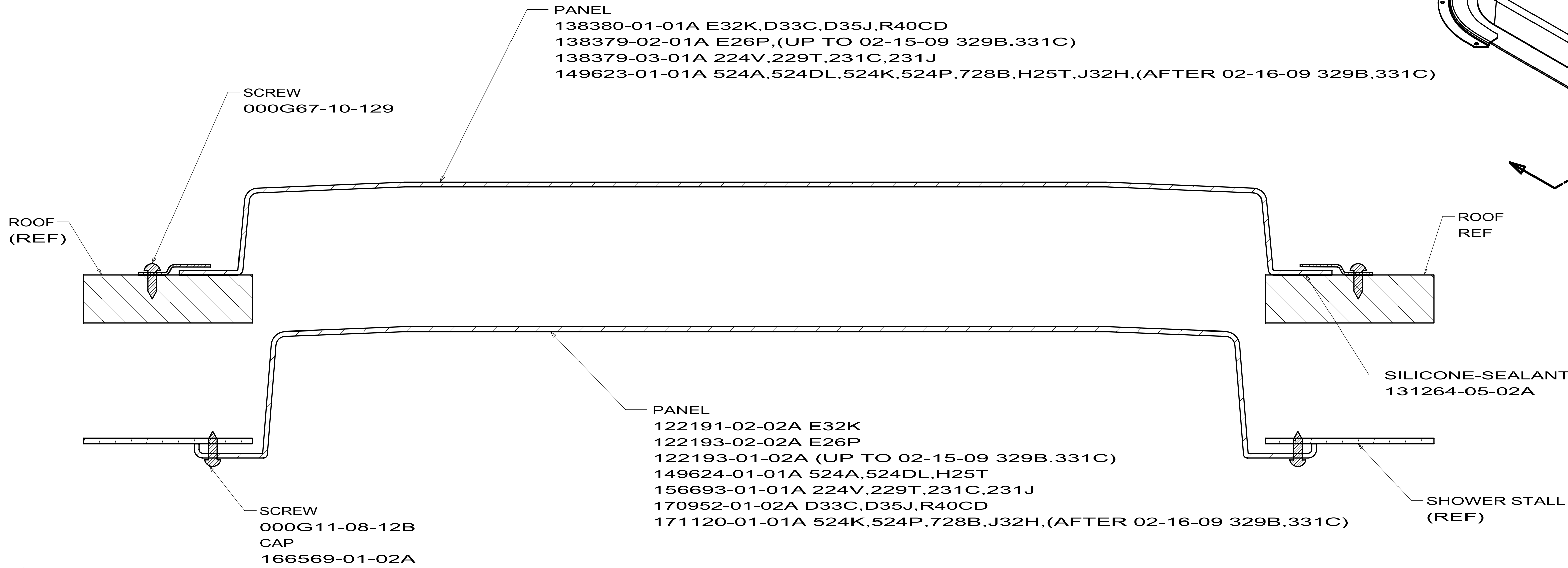
SECTION A-A
