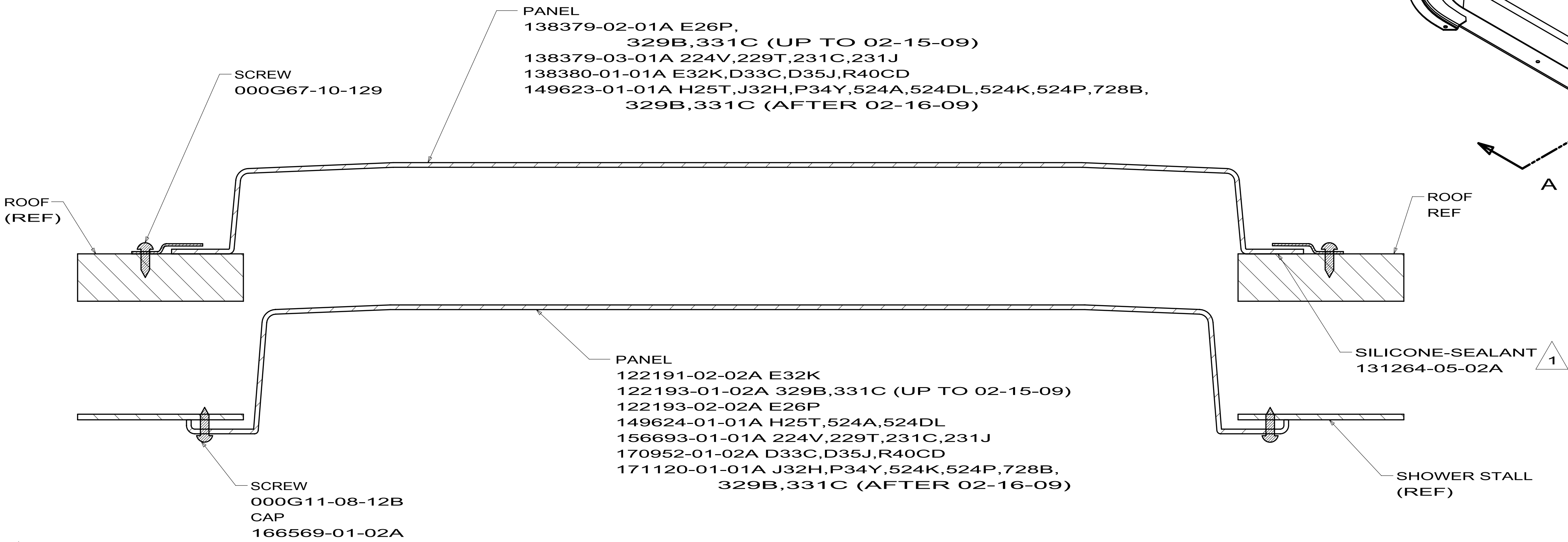
SECTION A-A
