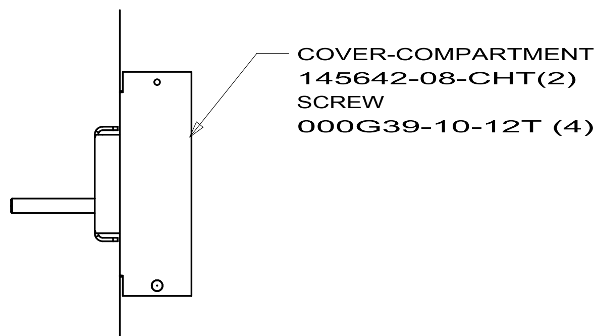
SECTION HJ-HJ
