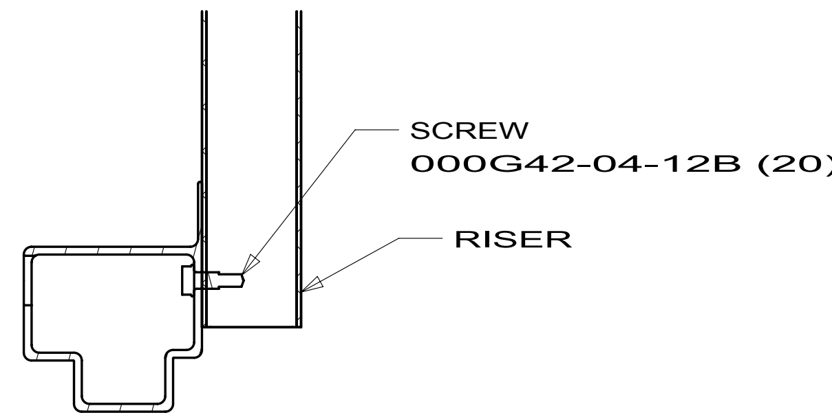
SECTION HD-HD
