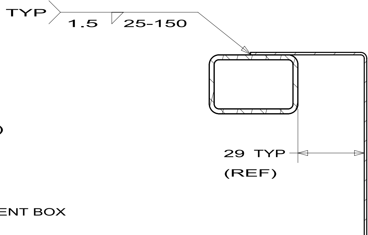
SECTION HC-HC
