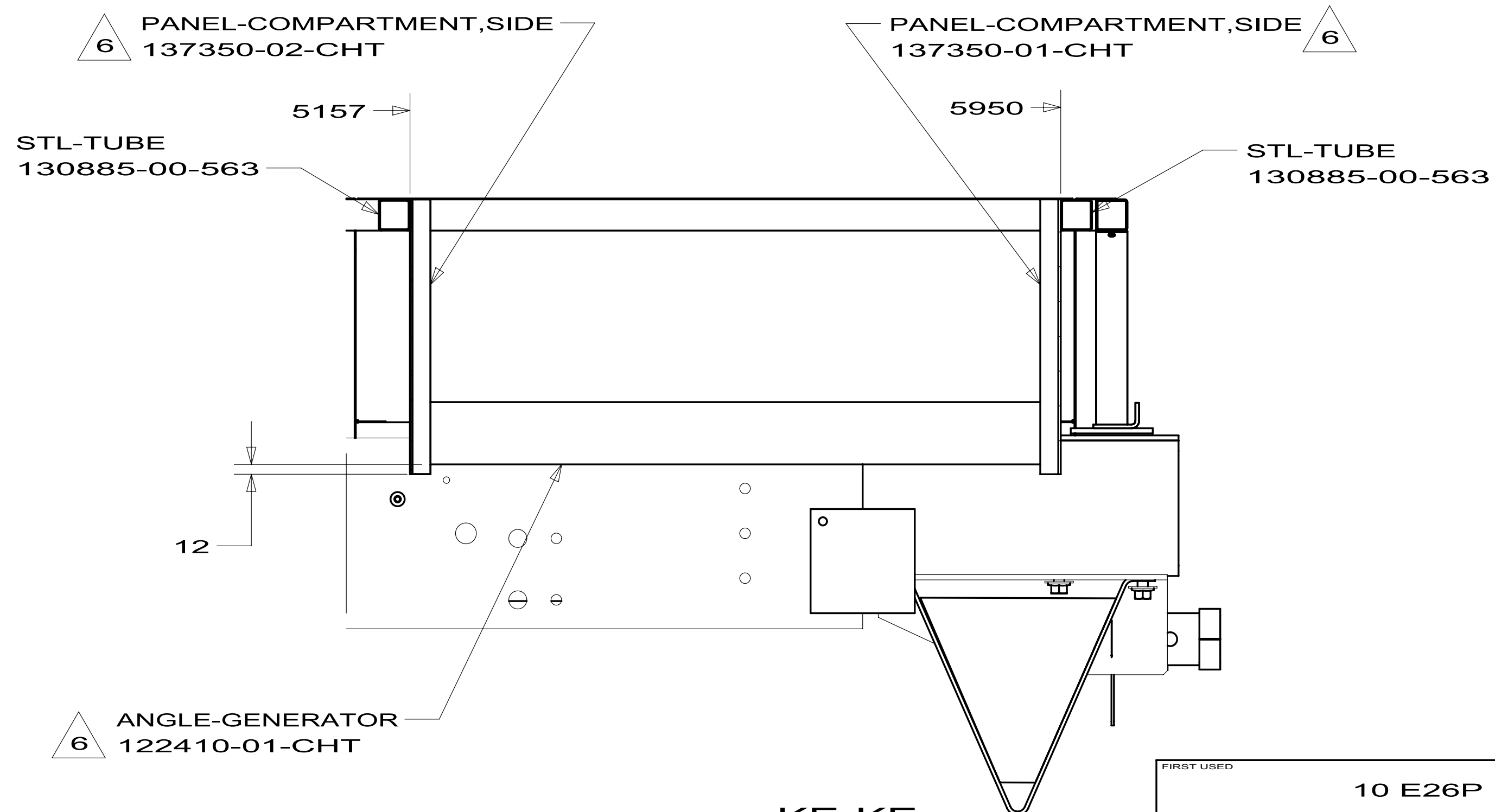
SECTION KE-KE
