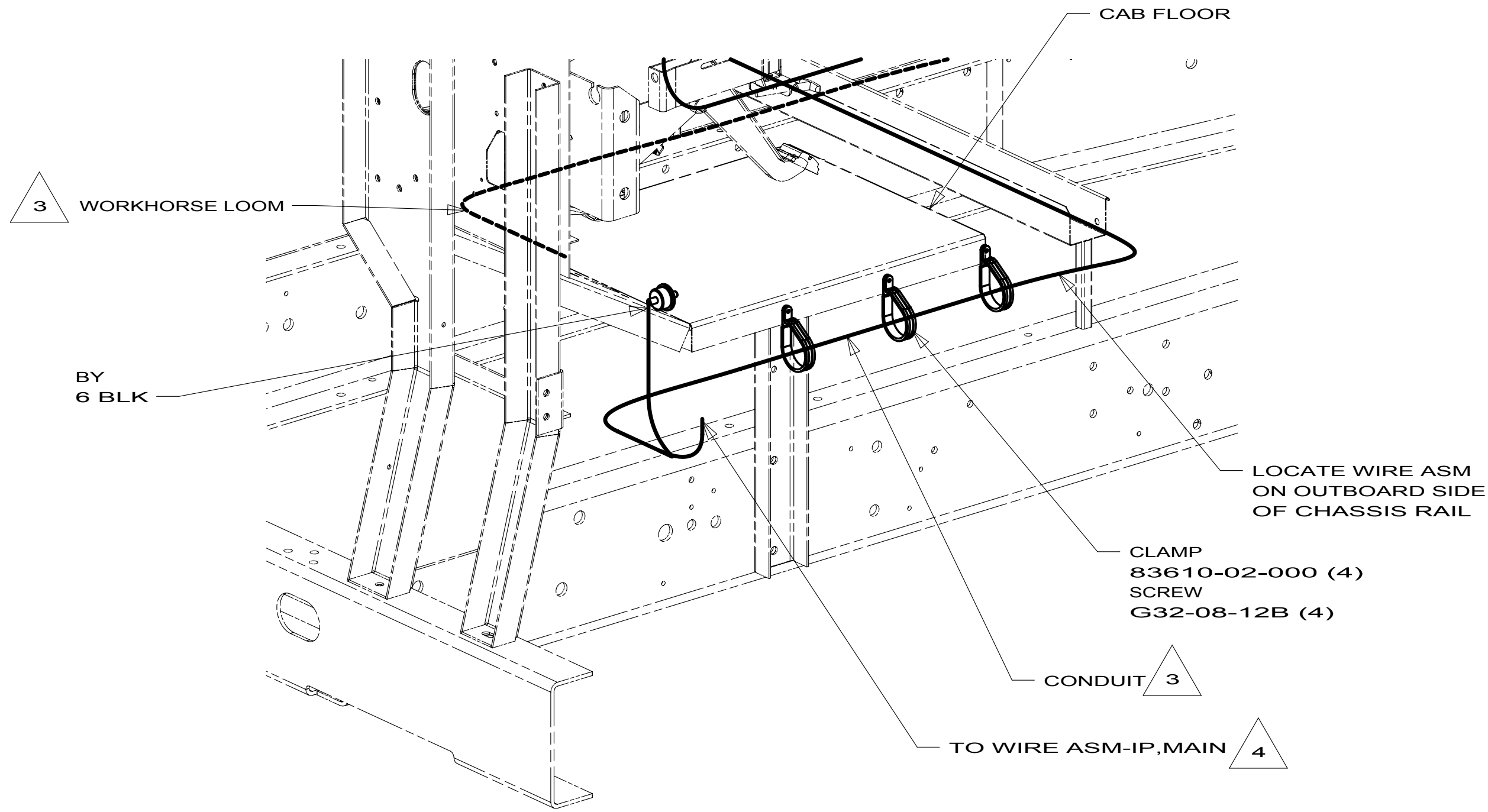
VIEW DA 1PS 1PU
