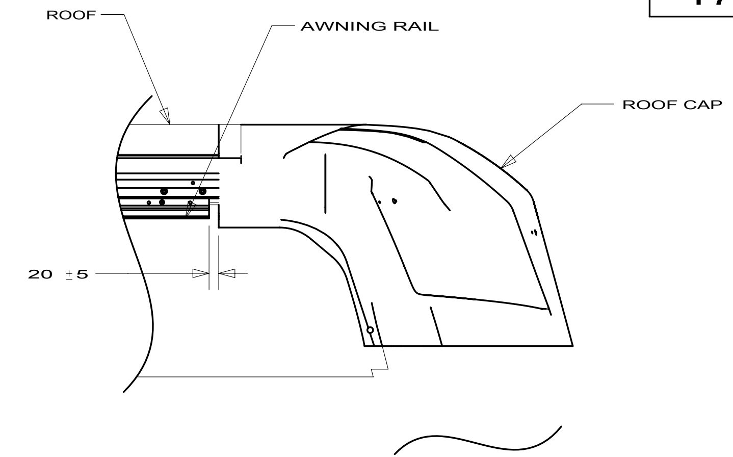
DETAIL AJ-AJ
