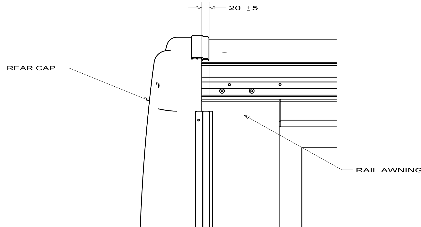
VIEW AK-AK
