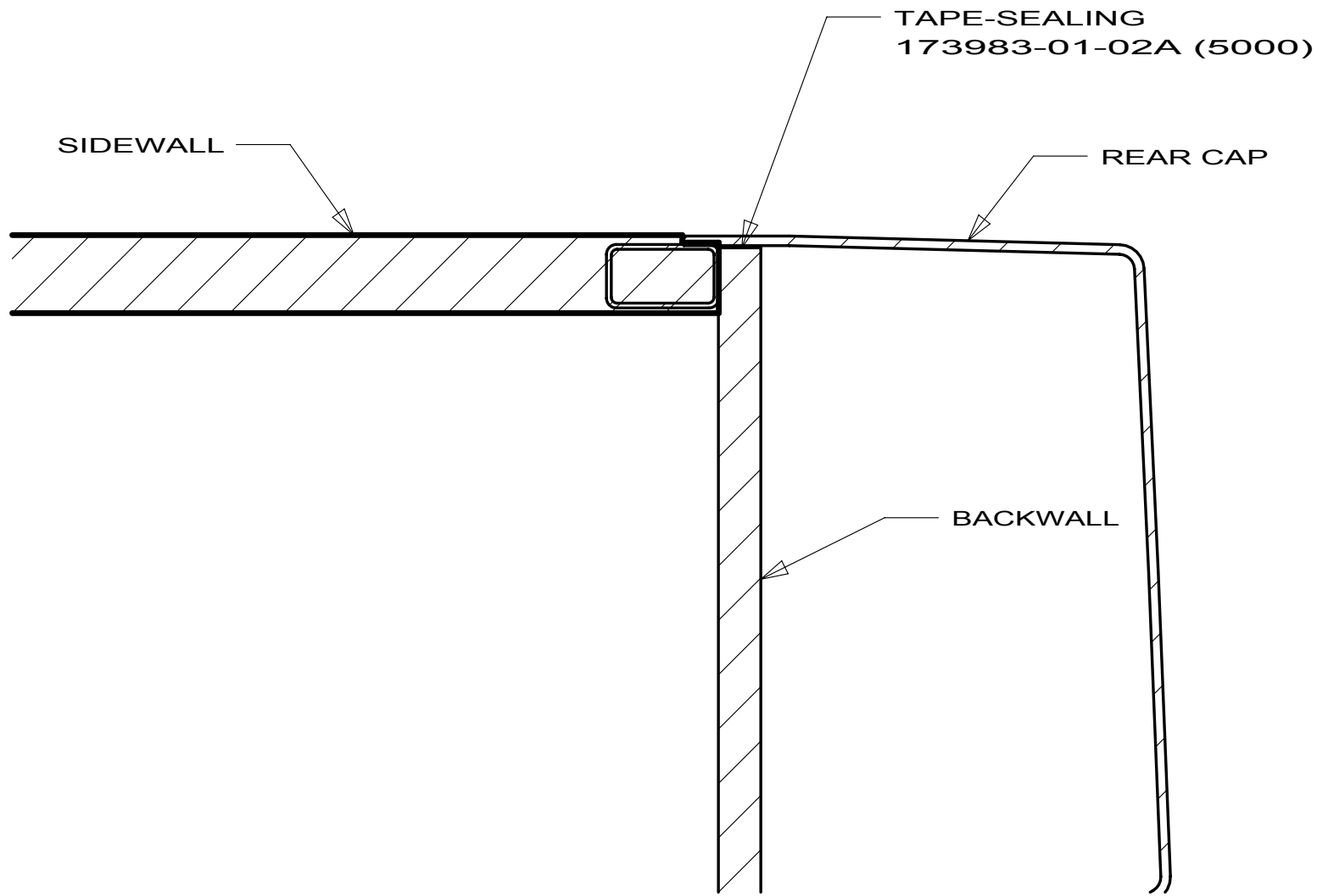
SECTION AK-AK
