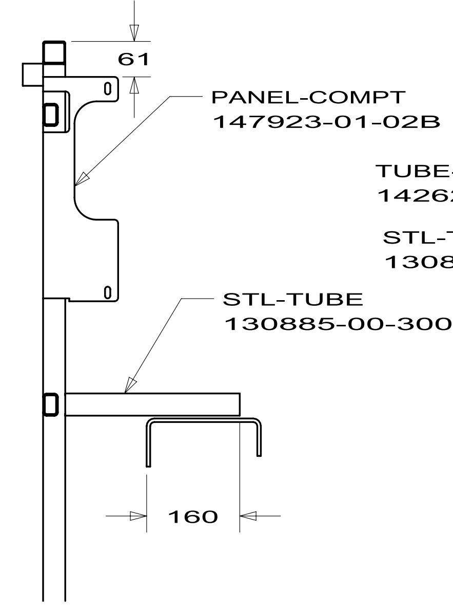
SECTION EK-EK
