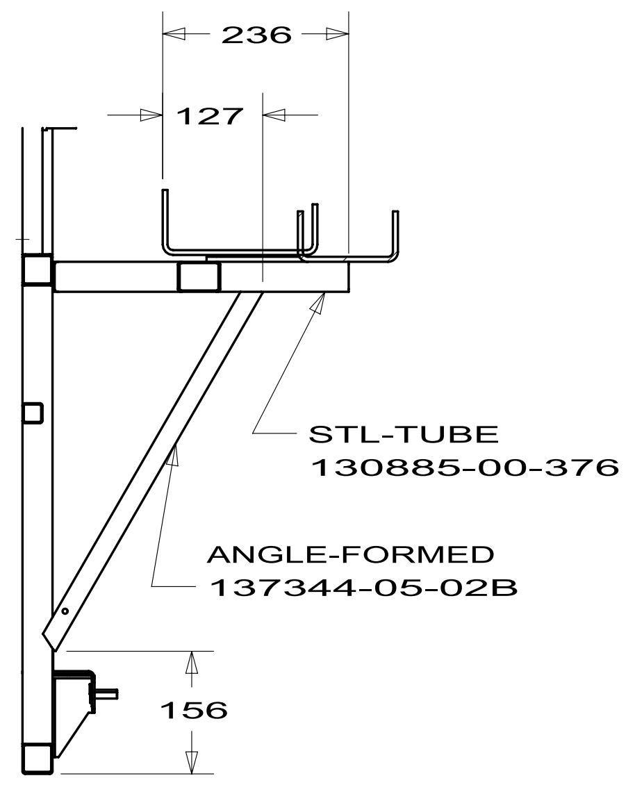
SECTION EF-EF
