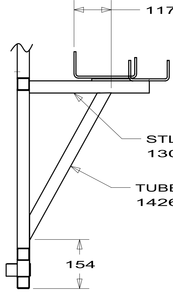
SECTION EH-EH (4 PLCS)
