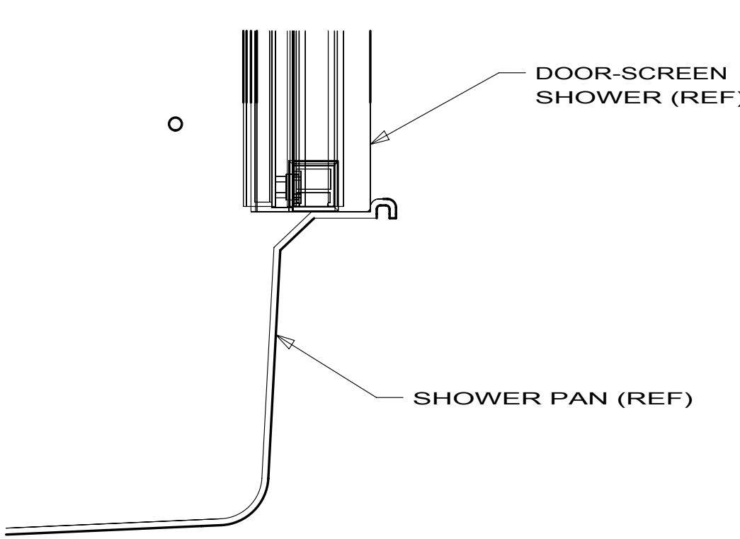
SECTION D-D
