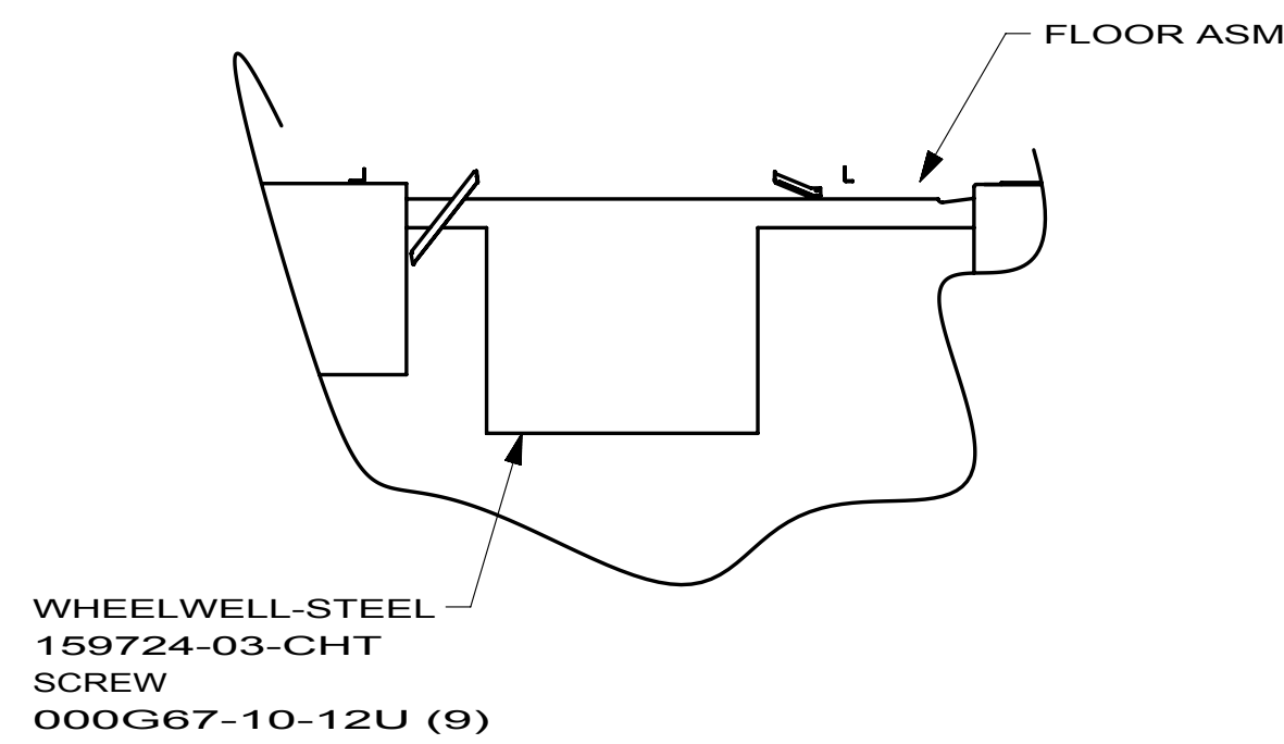
VIEW AK-AK
