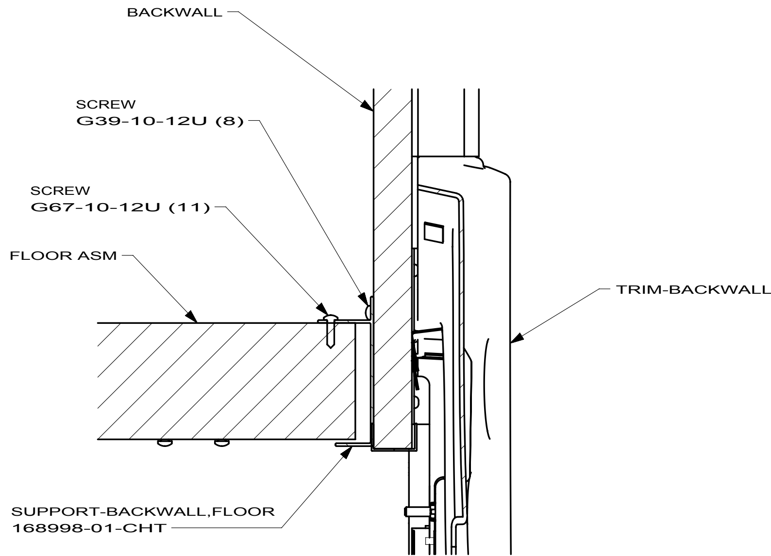
SECTION AA-AA
