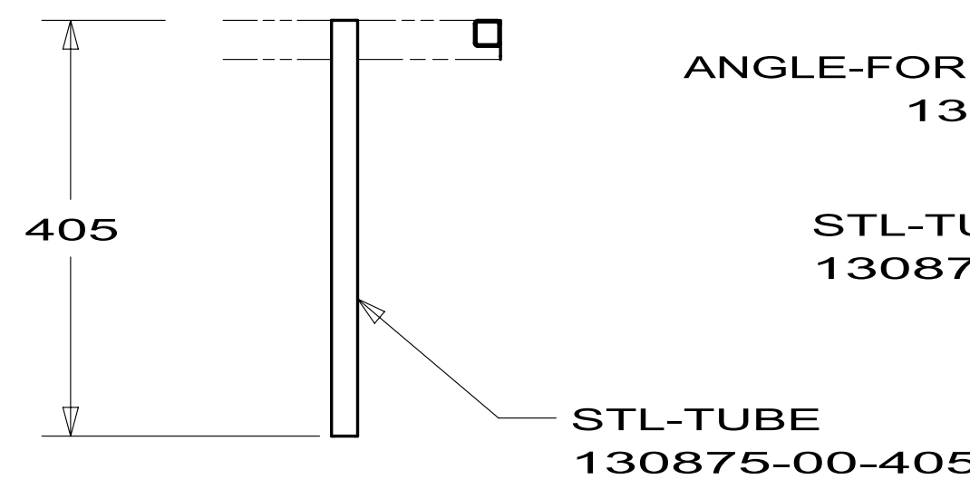
SECTION GL-GL
