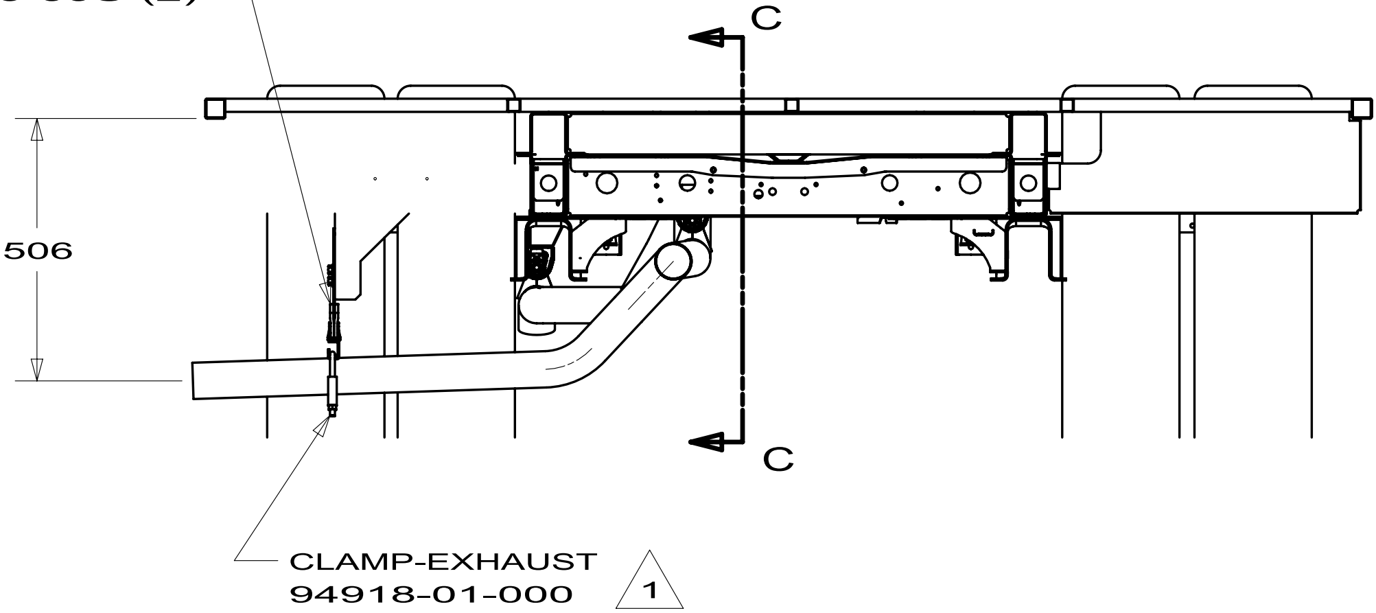
SECTION D-D
