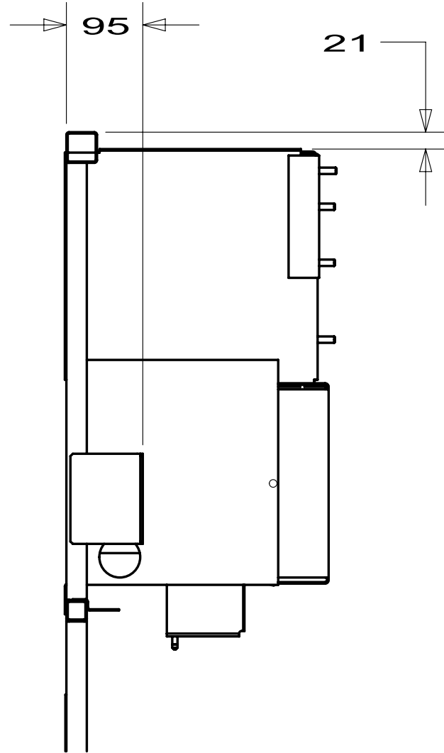
SECTION GA-GA
