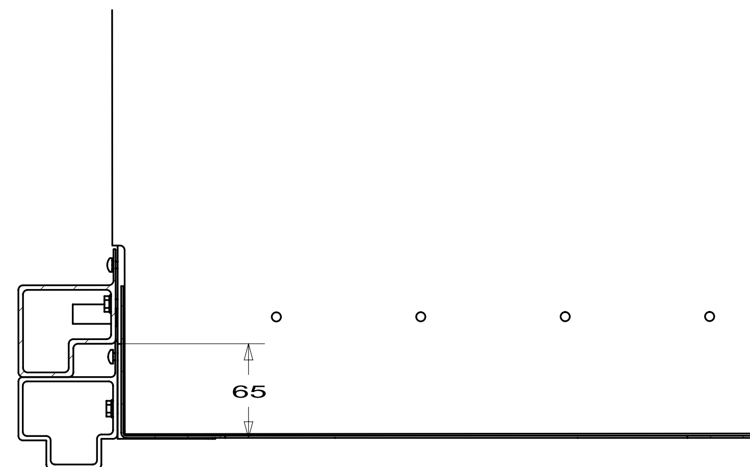
SECTION FE-FE
