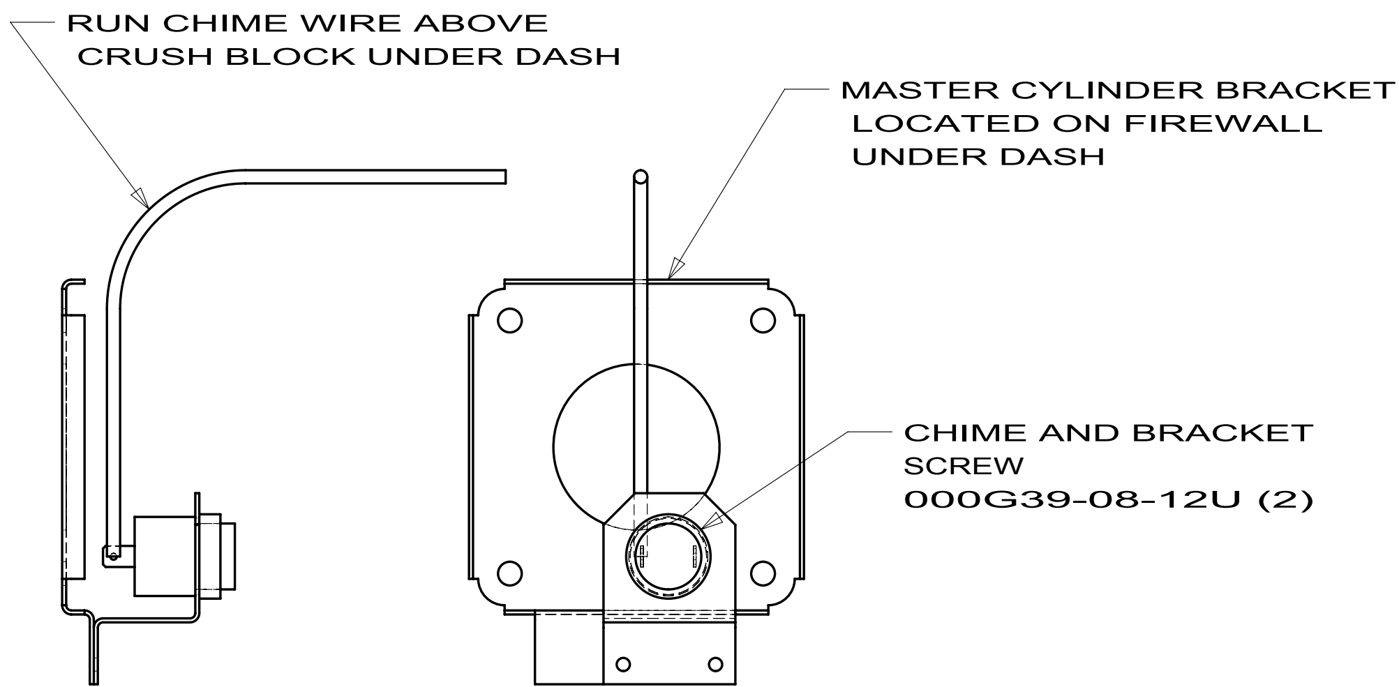
VIEW A-A
