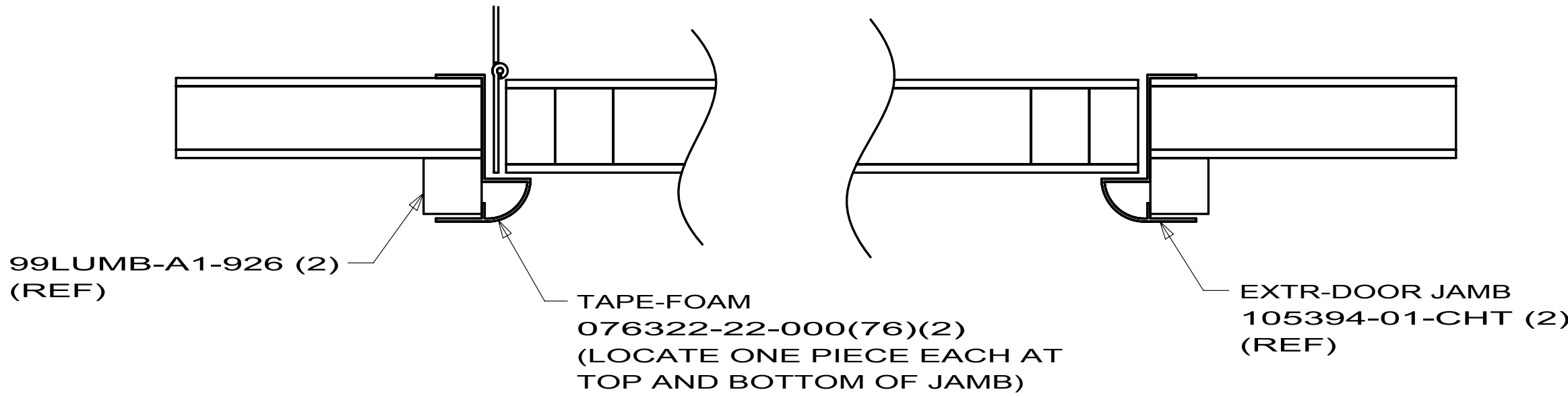
SECTION AJ-AJ
