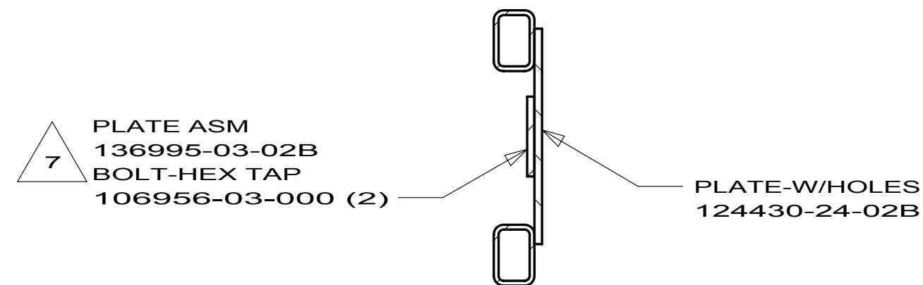
SECTION DD-DD 2 PLCS
