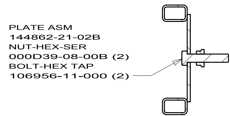
SECTION DC-DC 2 PLCS
