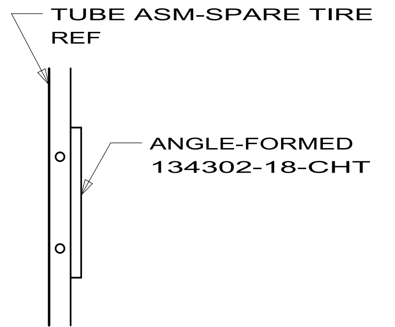
SECTION CD-CD
