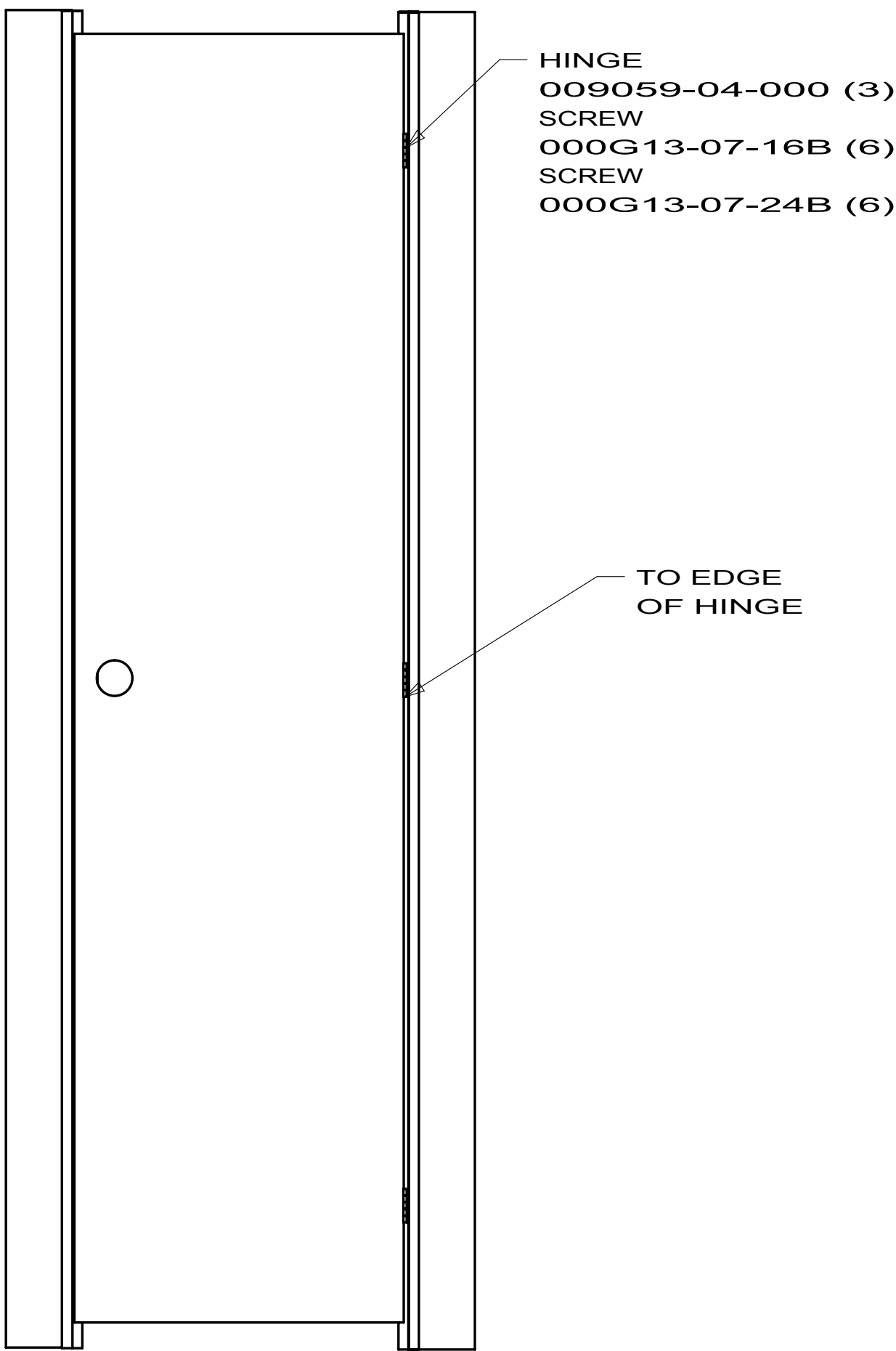
VIEW AZ
