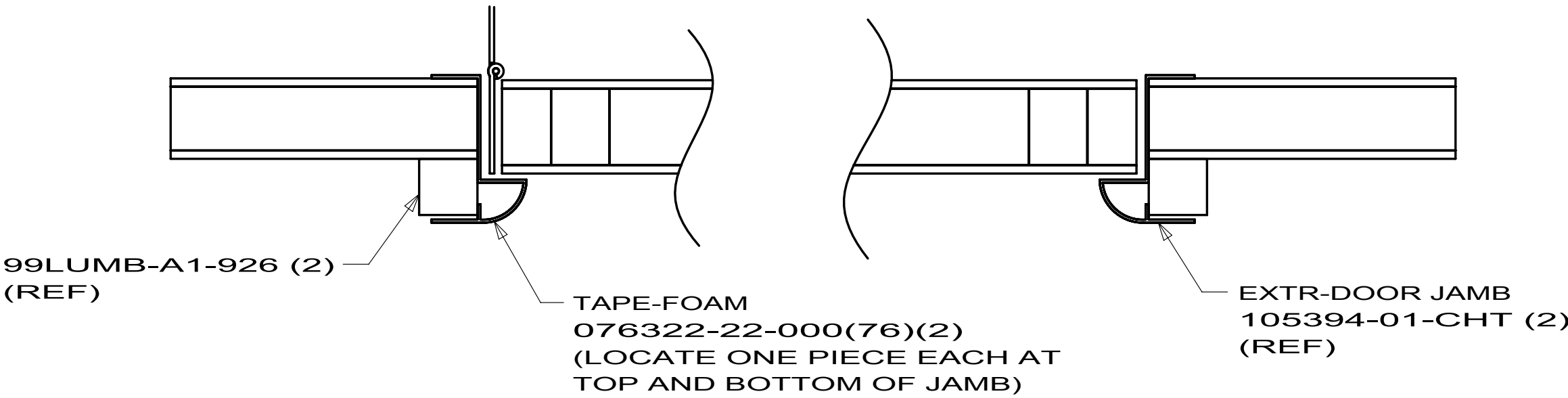
SECTION AJ-AJ
