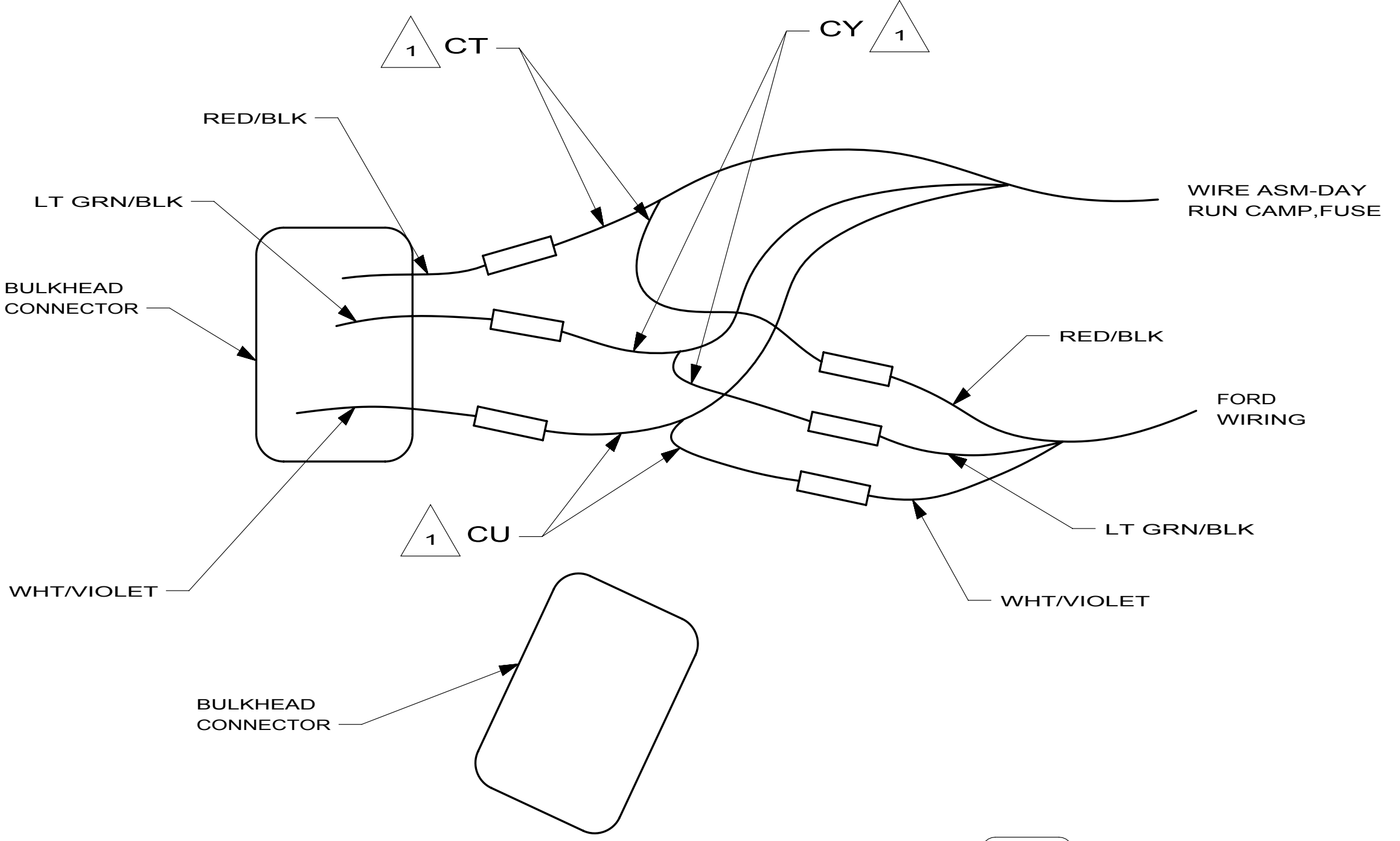
VIEW A-A
