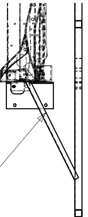
SECTION EM-EM
