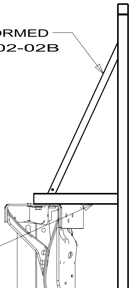
SECTION EK-EK
