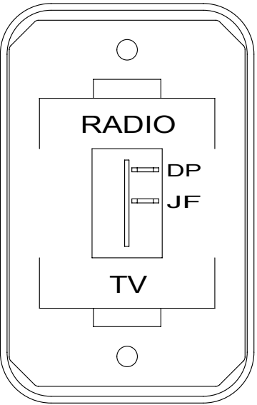
DETAIL CE 1JL
