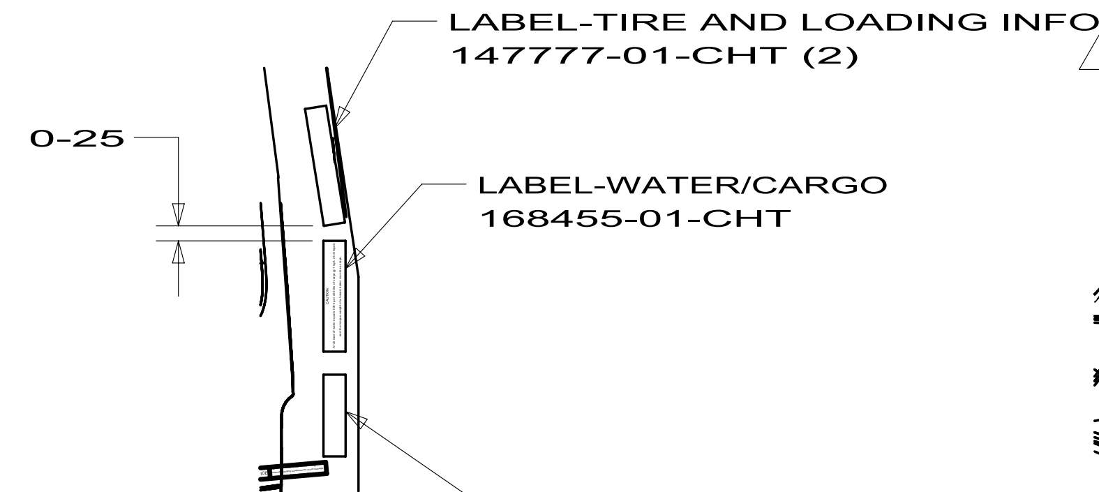
SECTION D-D
