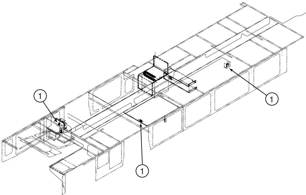
110V WIRING
