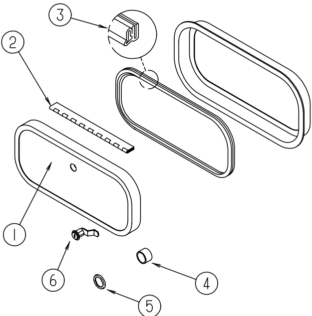
ENTERTAINMENT CENTER DOOR
