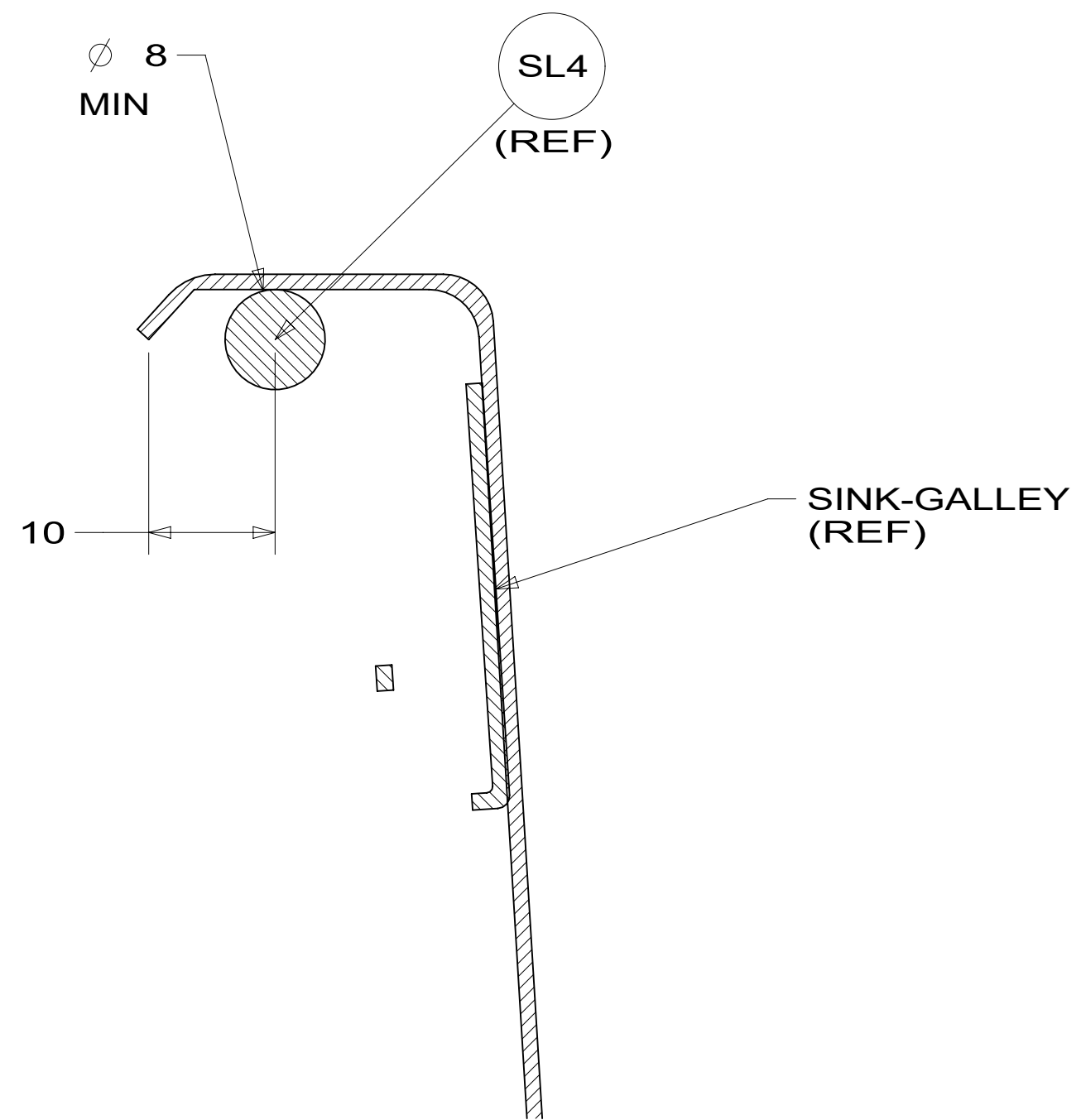
SECTION CE-CE
