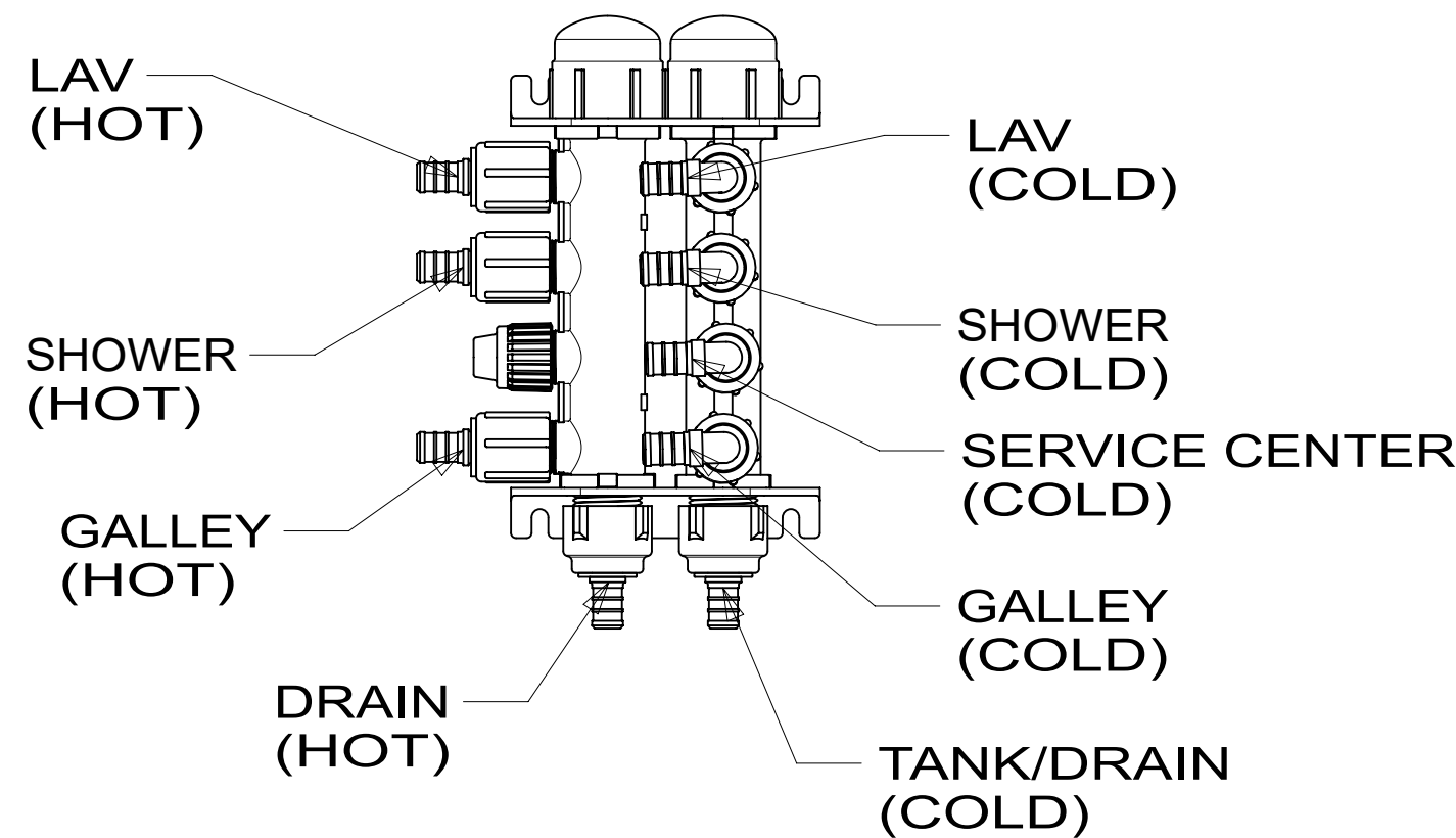
SECTION AA-AA
