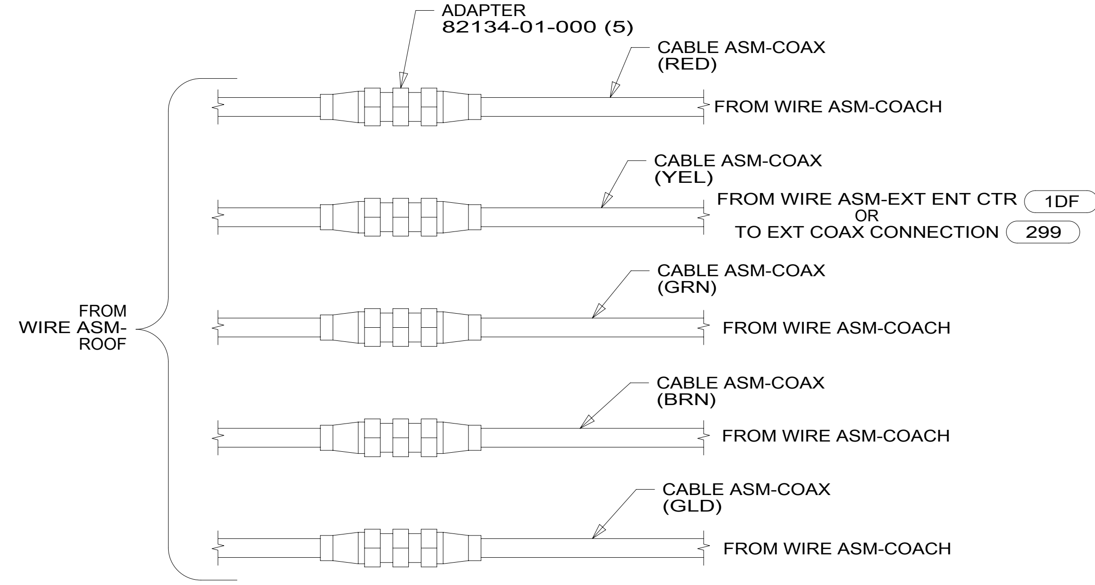
DETAIL DS
