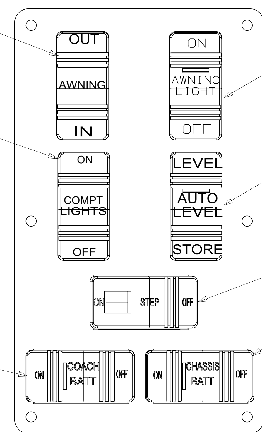
DETAIL DH
