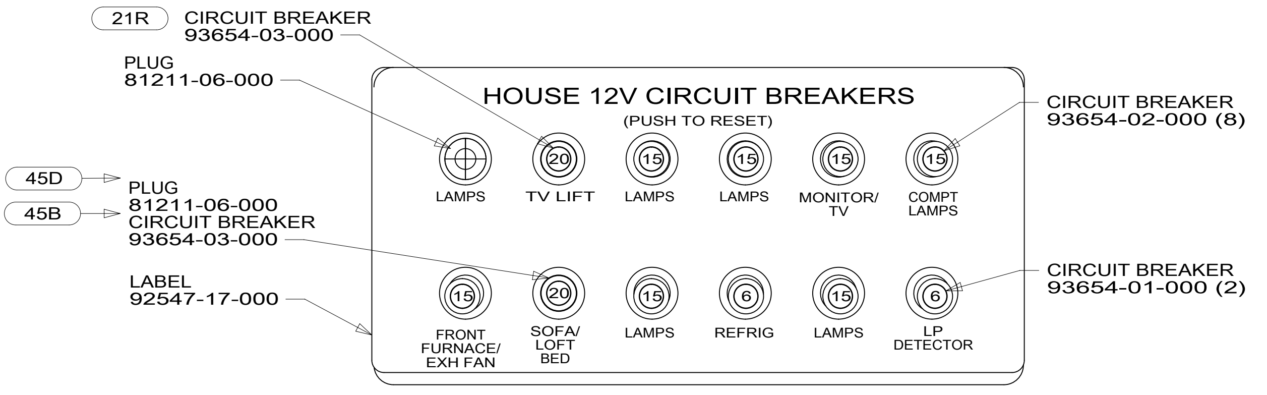
DETAIL DS 078 (FRONT VIEW)
