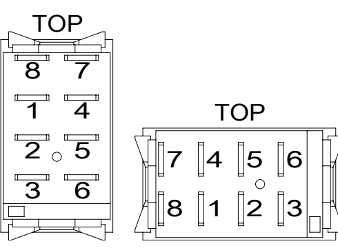
DETAIL DE
