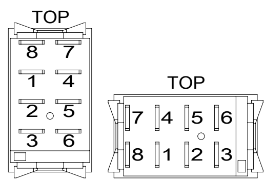
DETAIL DE
