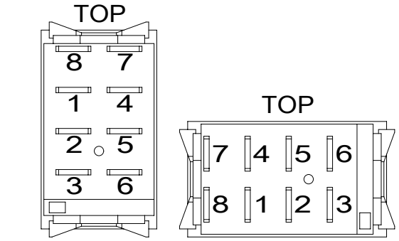
DETAIL EK
