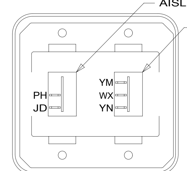
DETAIL EL
