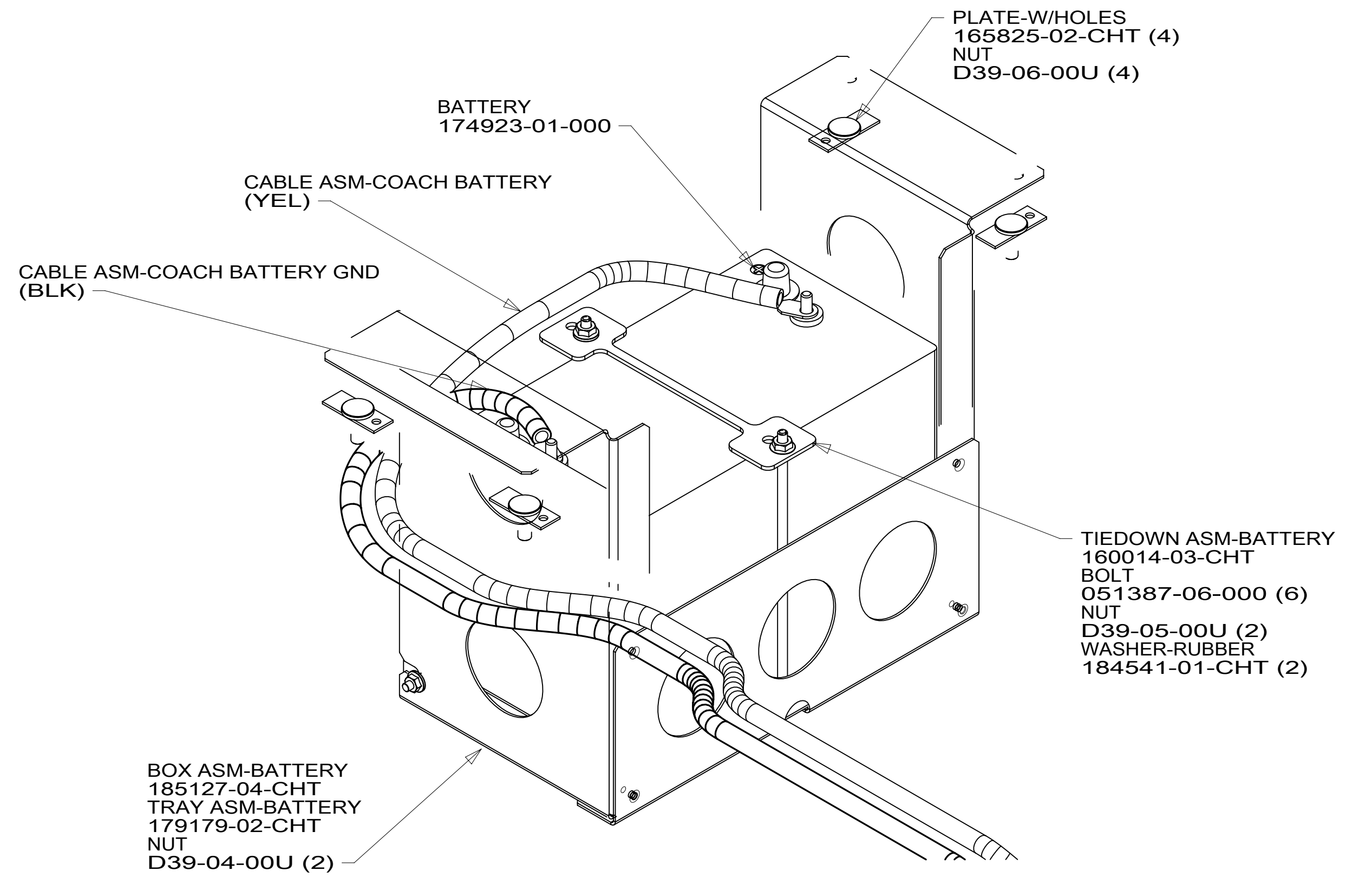
VIEW DA
